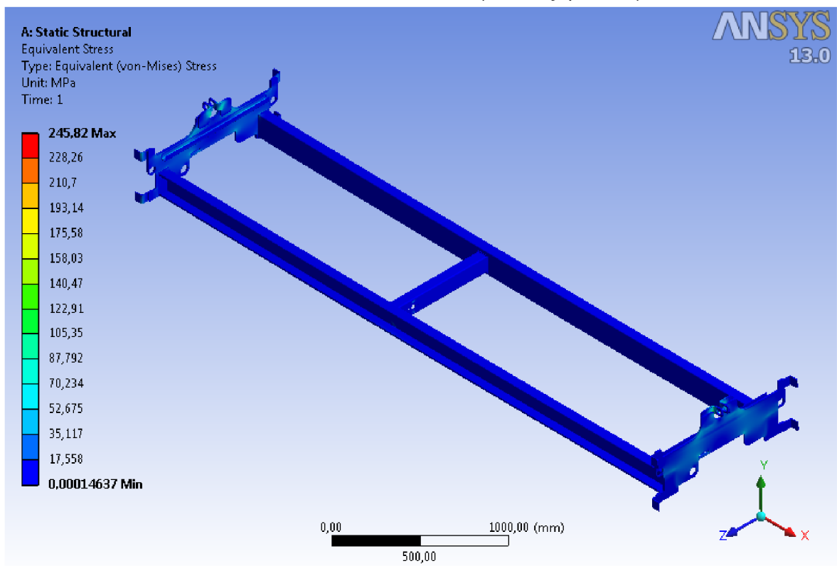
Obr. 22 Výsledky redukovaného napětí HMH (celkový pohled)
