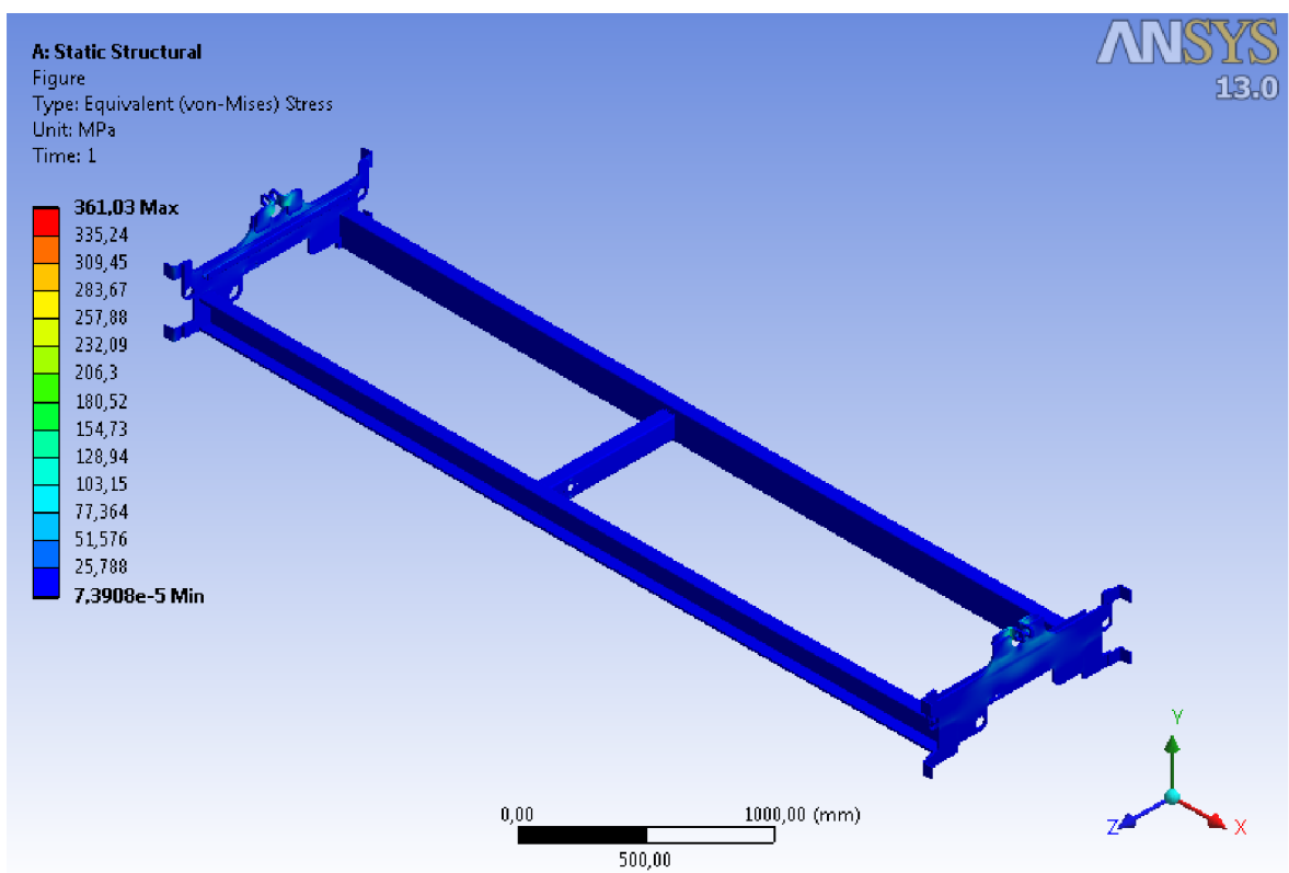
Obr. 31 Výsledky redukovaného napětí HMH (celkový pohled)
