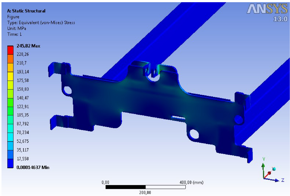
Obr. 37 Průběh redukovaného napětí HMH na bočnici 2
