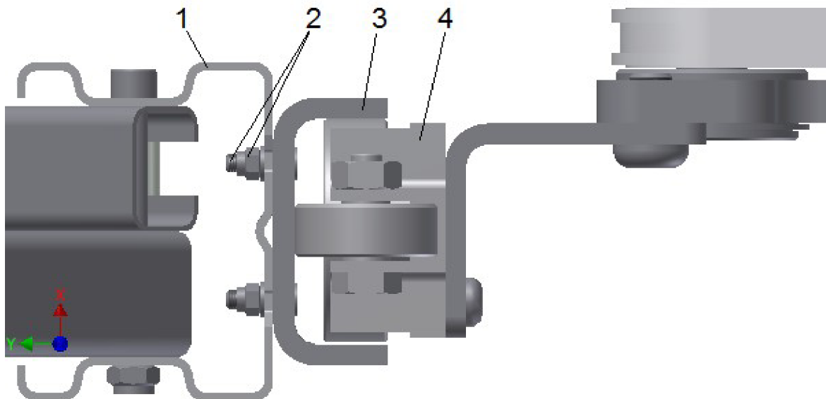
Obr. 39 Vedení elevátoru v rámu systému Logimat (1), šroubové spojení vodícího profilu s rámem (2), vodící profil (3), kombinovaná kladka (4)
