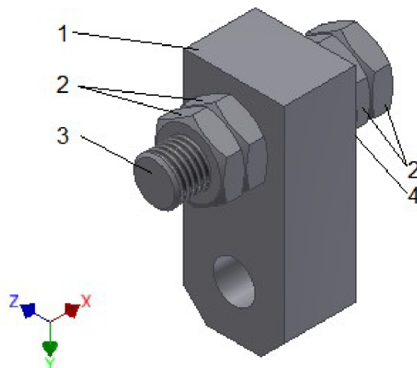
Obr. 16 Detail úchytu řetězu volné větve, spojovací kostka (1), matice ISO 4035 - M16 (2), závitová tyč M16 (3), podložka ISO 7089 - 16 - 140 HV (4)
