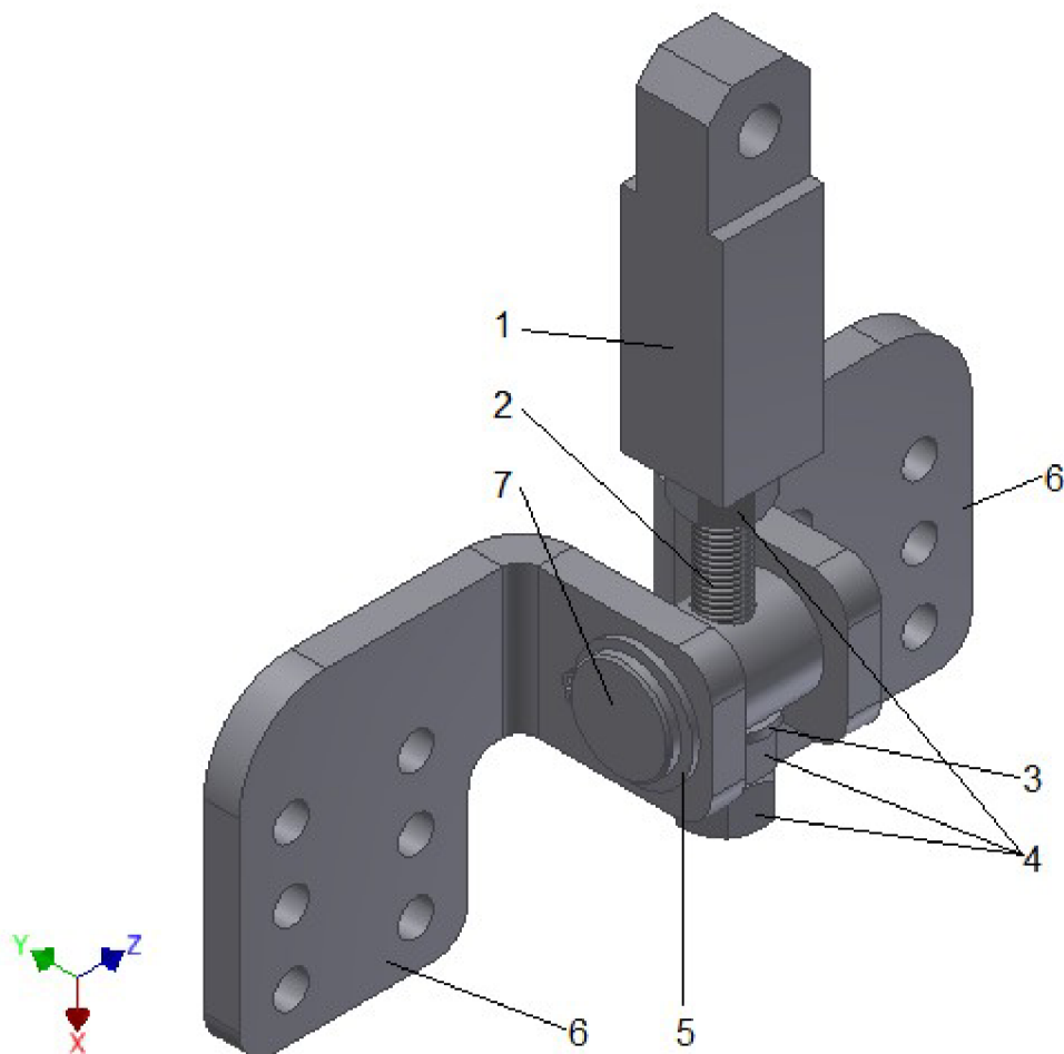
Obr. 17 Detail úchytu řetězu nosné větve, spojovací kostka (1), závitová tyč M16 (2), podložka ISO 7089 - 16 - 140 HV (3), matice ISO 4032 - M16 (4), pojistný kroužek DIN 471 - 35 x 2,5 (5), L packy uložení čepu (6), nosný čep (7)
