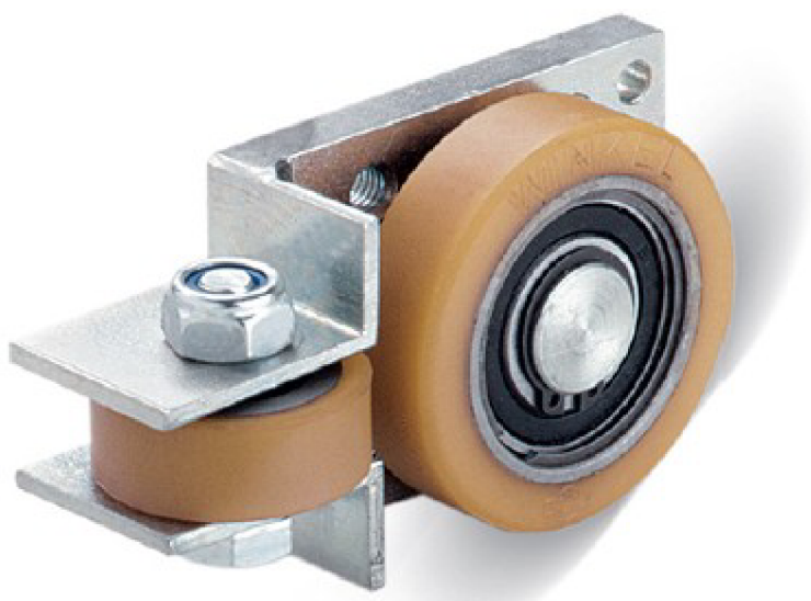
Obr.6 Kombinovaná kladka Vulkolan V6250AP [25]
