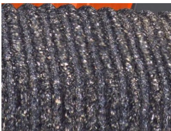
Obrázek 14: Profil mikrozávitů vyfocený pomocí 3D Zeiss mikroskopu na Mezinárodním strojírenském veletrhu
