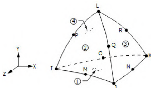
Obrázek 28: Prvek kvadratického čtyřstěnu SOLID 187
