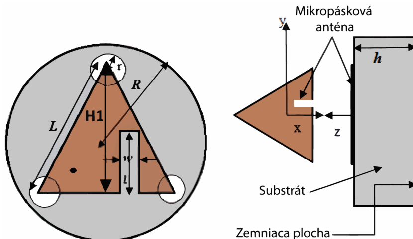
Obr. 2.1: Nákres antény prebratý a preložený z [1].
