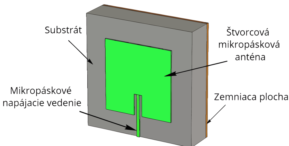
Obr. 1.1: Príklad mikropáskovej antény s mikropáskovým napájacím vedením.
