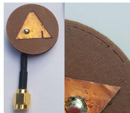
(b) Anténa s detailným pohľadom na vzniknuté dierky.
