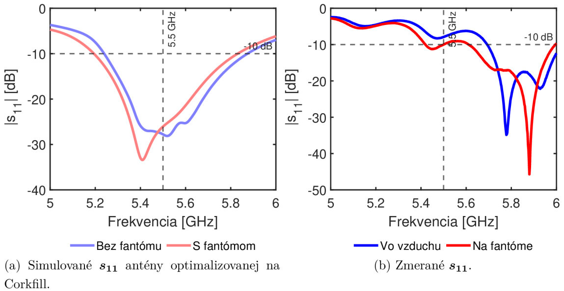
Obr. 3.6: Grafy najlepších hodnôt s_{11} pre materiál corkfill.
