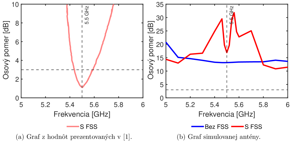
Obr. 2.11: Graf osového pomeru pôvodnej antény (osi y majú rôzny rozsah!).
