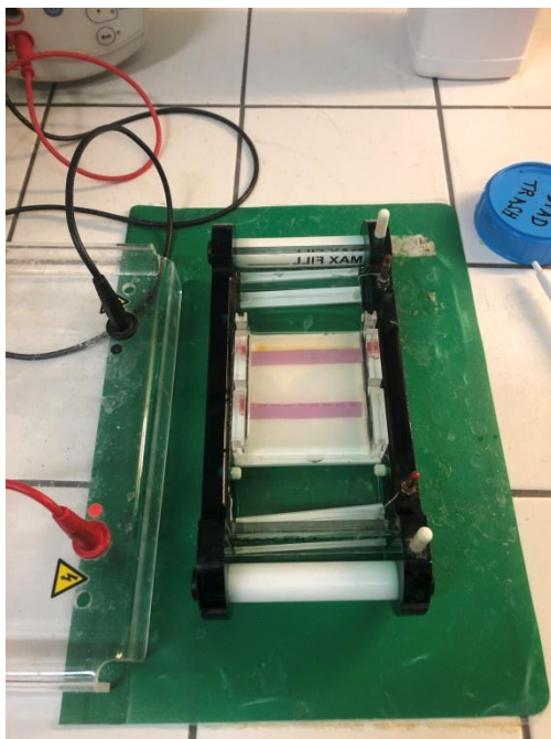
Obr. 20. Elektroforeza
