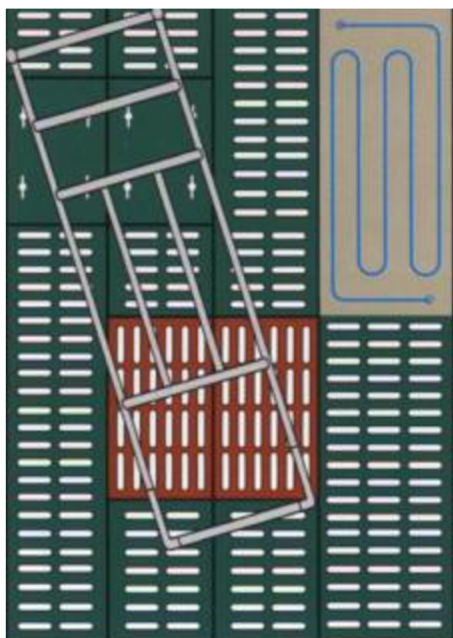
Obrázek 1 Návrh porodního kotce (Stupka et al., 2013)
