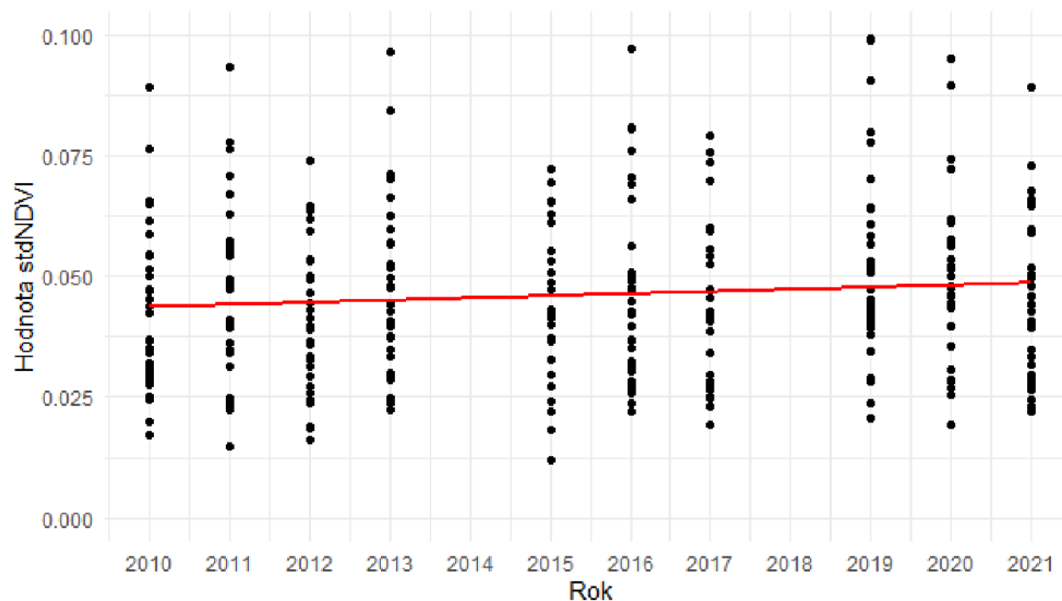
Obrázek 59. Graf lineární regrese pro rozlišení 7x7 směrodatné odchylky NDVI pro lokality zasažené mírnými požáry od 1998 do roku 2010 hodnoty jsou: R^2 = 0,009 , \beta = 0,00053 a p-hodnota = 0,05.
