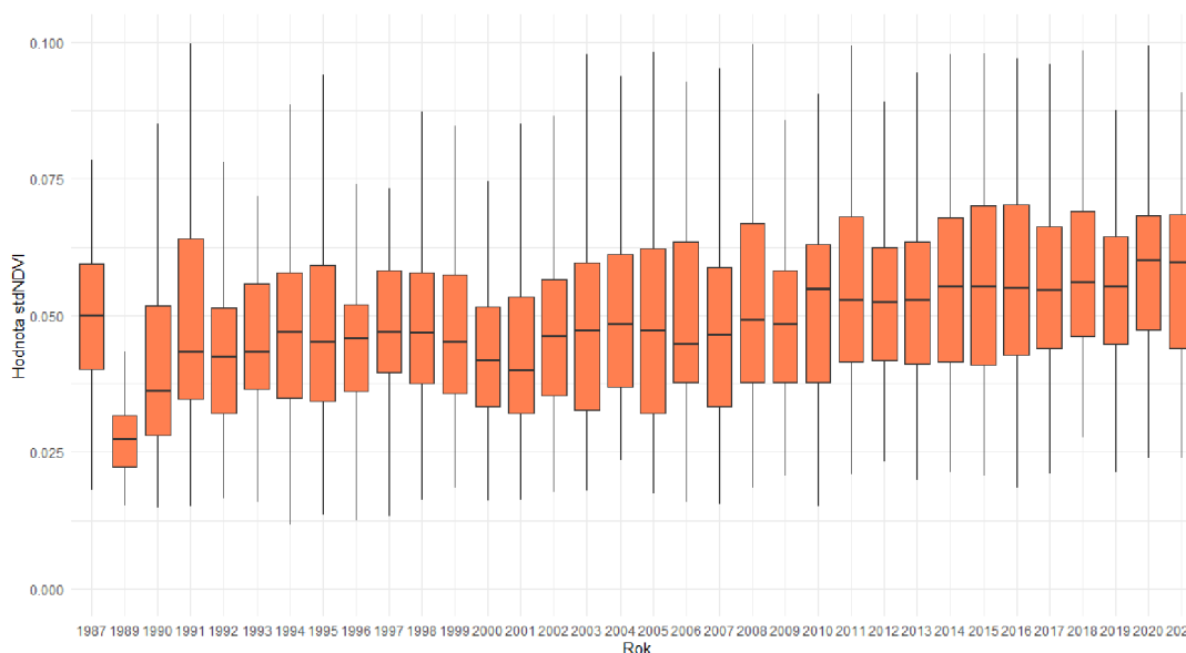
Obrázek 23. Rozsah hodnot a mediány ze směrodatné odchylky NDVI pro lokality zasažené požárem v roce 1988 v rozlišení 9x9.
