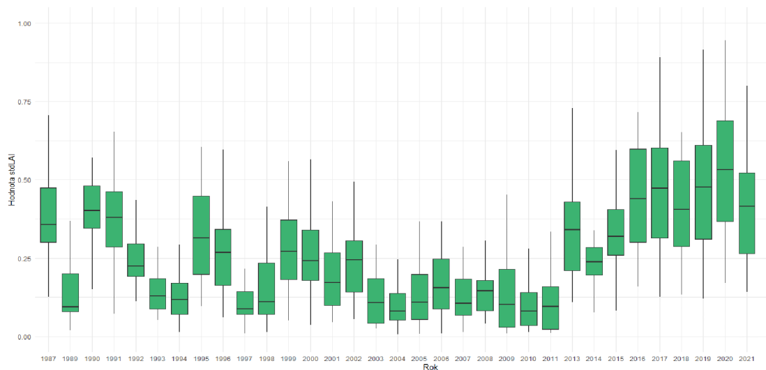
Obrázek 41. Rozsah hodnot směrodatné odchylky LAI v rozlišení 9x9.
