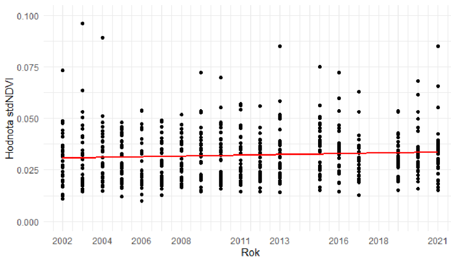
Obrázek 45. Vývoj lineární regrese směrodatné odchylky v rozlišení 5x5 od posledního požáru. R^2 = 0,009 , \beta = 0,0014 a p-hodnota = 0.001434
