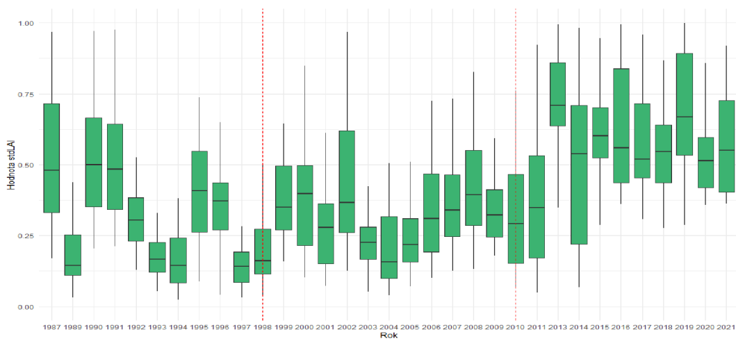
Obrázek 64. Rozsah hodnot směrodatné odchylky LAI v rozlišení 9x9.
