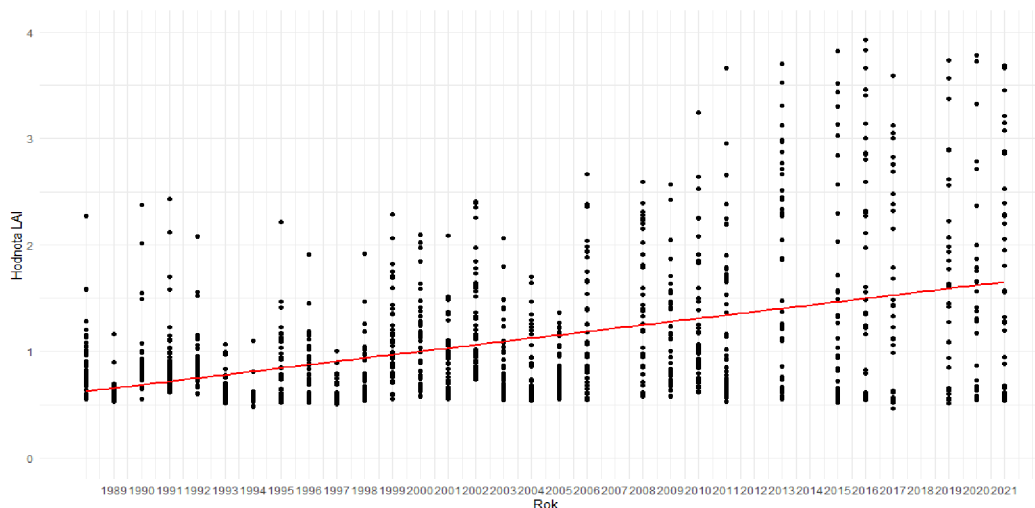
Obrázek 28. Lineární regrese pro index LAI pro lokalitu zasaženou požárem v r. 1988. Kde je R^2 = 0.2663 , \beta = 0.06226 a p < 0.001 .
