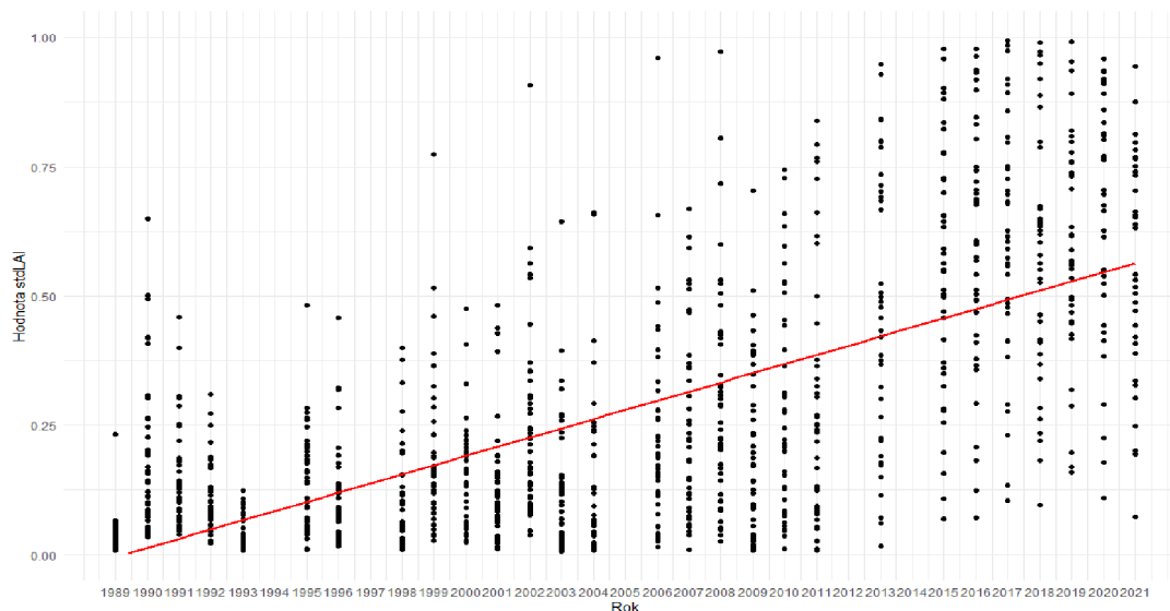
Obrázek 32. Graf lineární regrese spektrální variability STD v rozlišení 9x9 z LAI pro lokalitu zasaženou požárem v r. 1988.
