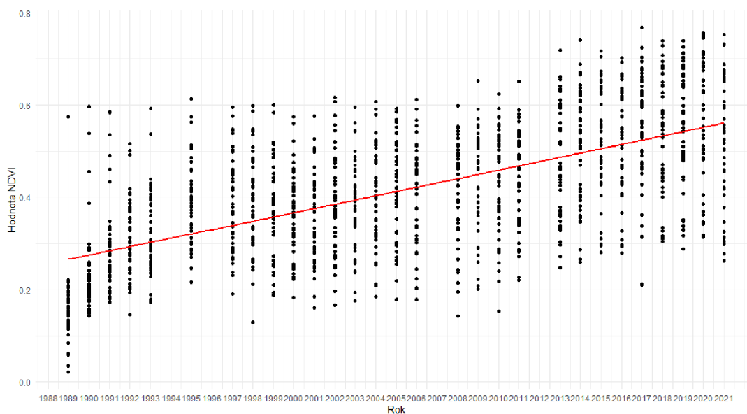
Obrázek 15. Graf lineární regrese pro NDVI od roku 1989. R^2 = 0,283 , \beta = 0,0762 a p < 0.001 .
