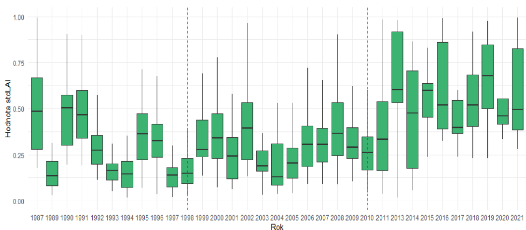
Obrázek 62. Rozsah hodnot směrodatné odchylky LAI v rozlišení 5x5.
