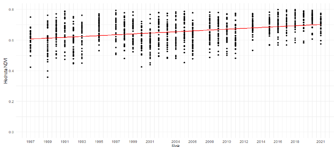
Obrázek 34. Lineární regrese pro NDVI na místech nezasážených požárem, kde R^2 = 0.163 , \beta = 0.0035 a p < 0.001 .
