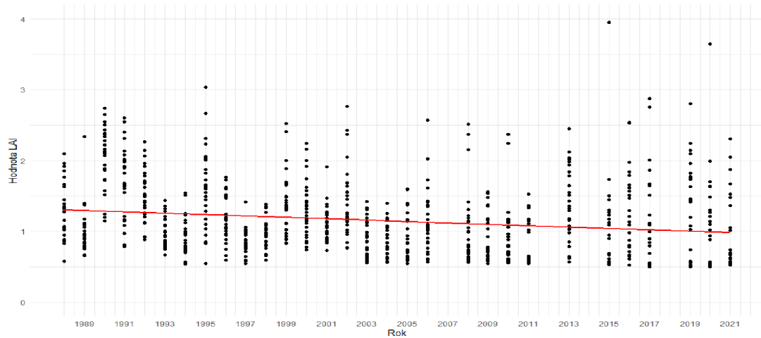
Obrázek 40. Lineární regrese pro index LAI pro lokalitu nezasazenou požárem. Kde je R^2 = 0.00004 , \beta = -0.00024 a p-hodnota = 0,9365.
