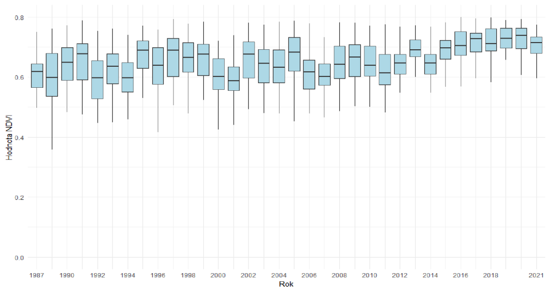
Obrázek 33. Hodnoty NDVI na místech nezasážených požárem.
