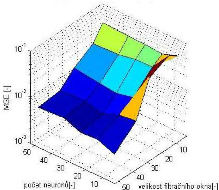
Obr. 20 Graf vývoje střední kvadratické chyby mse
