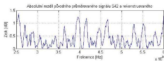
Obr. 29 Přichycení sítě k trénovacím vzorům (vlevo nahoře), absolutní odchylka původního a rekonstruovaného signálu (vpravo nahoře) a rozložení RBF jader (vlevo dole)
