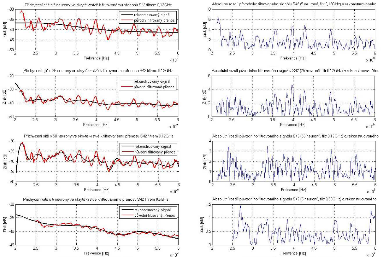
Obr. 11 Průběhy přichycení sítě k filtrovanému přenosu S42 a vzájemný rozdíl pro několik různých architektur sítě a velikostí průměrovacího okna
