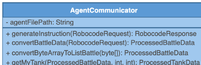
Obr. 3.6: UML diagram třídy AgentCommunicator
