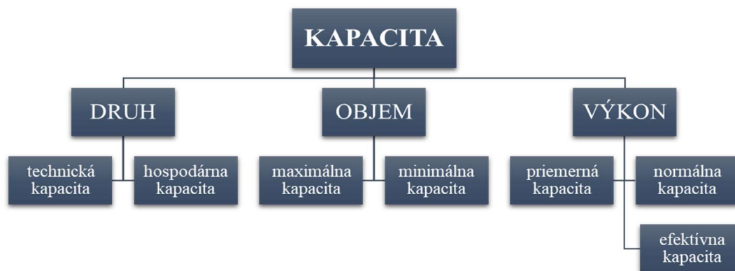
Obr. 4) Klasifikácia kapacít [14]
