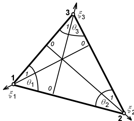
Obr. 3.7 Dvojrzměrné simplexní souřadnice.
