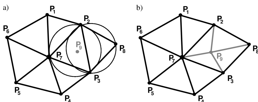
Obr. 3.3 Bowyerův-Watsonův algoritmus pro generování Delaunayho trojúhelníkové sítě: a) testování opsanými kružnicemi, b) zjemnění sítě.
