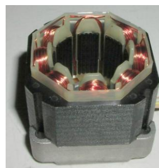
Obrázek 3.1 Stator KM [3]
