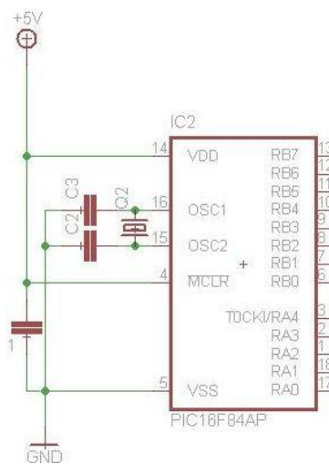
Obrázek 5.5 Realizace krystalového oscilátoru
