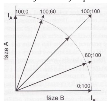
Obrázek 3.22 Mikrokrokování
