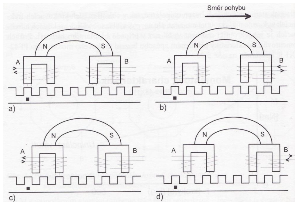
Obrázek 3.13 Princip Sawyerova lineárního motoru [2]
