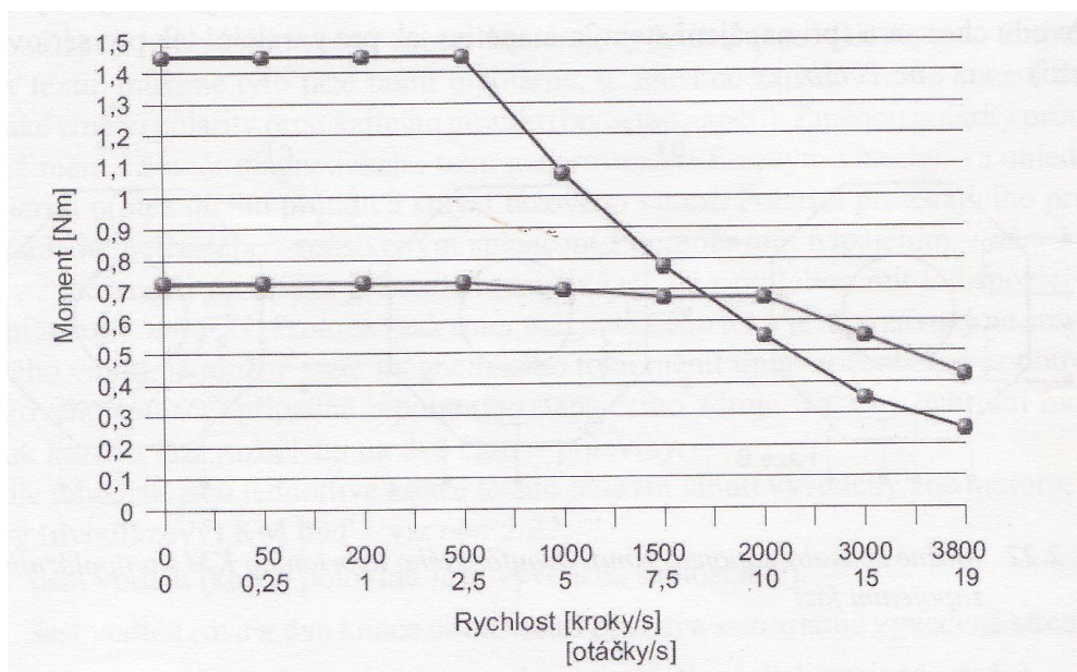
Obrázek 3.12 Momentová charakteristika motoru SX34-2740 (sériové zapojení – horní průběh, paralelní zapojení dolní průběh) [2]
