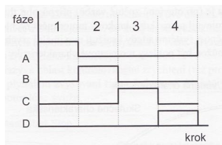
Obrázek 3.17 Čtyřtaktní řízení s magnetizací jedné fáze
