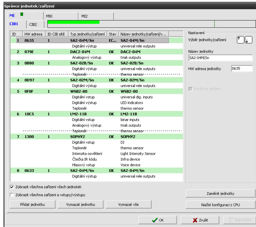
Obr. 3-3 „Správce jednotek/zařízení“.
