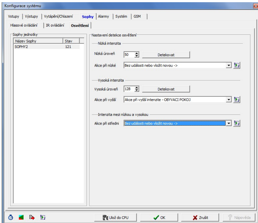
Obr. 3-16 „Konfigurace systému“, Sophy/osvětlení.
