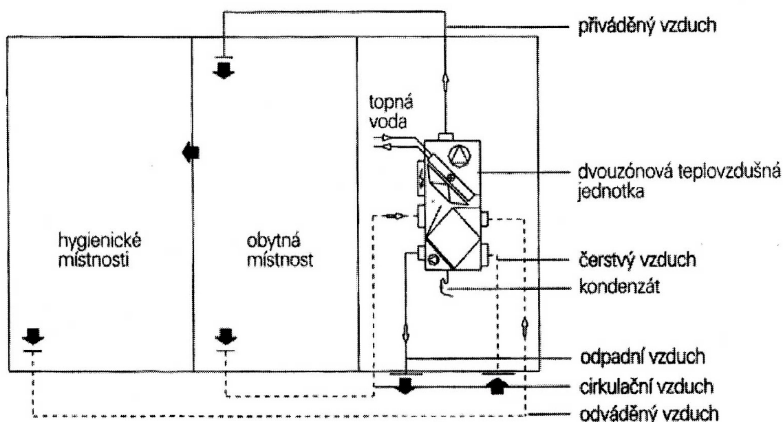
Obr. 3.1 Schéma dvouzónového tepl vzdušného vytápění [1]
