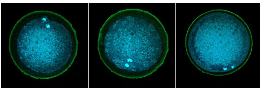
Obrázek 10. Lokalizace vybraných sacharidových struktur na zoně pellucidě u oocytů ve stádiu MII pomocí lektinu WGA. Biotinem značený WGA lektin se specificky váže na N-acetylglukosamin a N-acetylneuraminové kyseliny. WGA je na snímcích označen zeleně. Barvivo DAPI značí modrou barvou chromatin. Oocyty byly snímány konfokálním mikroskopem se zvětšením 400x.
