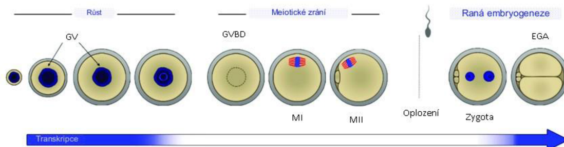
Obrázek 2. Schéma oogeneze a časného vývoje myšního embrya. Modrá šipka znázorňuje transkripční aktivitu. Na obrázku je zobrazený zárodečný váček (GV), rozpad zárodečného váčku (GVBD), oocyt v metafázi prvního meiotického dělení (MI), v metafázi druhého meiotického dělení (MII), zygota a EGA neboli embryo s aktivovaným embryonálním genomem (převzato a upraveno dle Christou-Kent et al. 2020).
