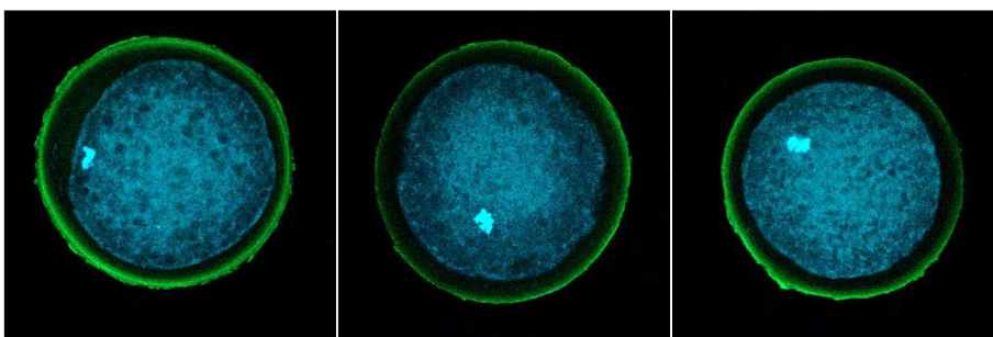
Obrázek 9. Lokalizace vybraných sacharidových struktur na zoně pellucidě u oocytů ve stádiu MI pomocí lektinu WGA. Biotinem značený WGA lektin se specificky váže na N-acetylglukosamin a N-acetylneuraminové kyseliny. WGA je na snímcích označen zeleně. Barvivo DAPI je modrou barvou a označuje chromatin. Oocyty byly snímány konfokálním mikroskopem se zvětšením 400x.
