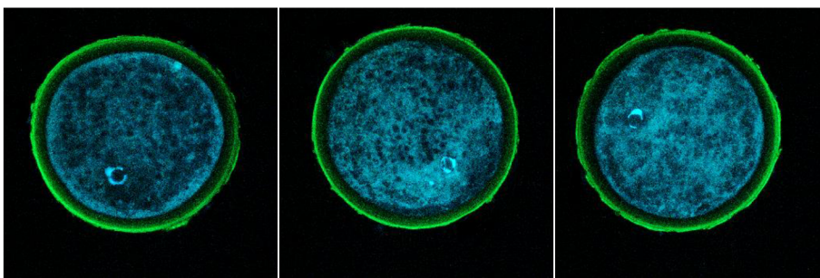
Obrázek 8. Lokalizace vybraných sacharidových struktur na zoně pellucidě u oocytů ve stádiu GV pomocí lektinu WGA. Biotinem značený WGA lektin se specificky váže na N-acetylglukosamin a N-acetylneuraminové kyseliny. WGA je na snímcích označen zeleně. Modrou barvou je označen chromatin pomocí barviva DAPI. Oocyty byly snímány konfokálním mikroskopem se zvětšením 400x.
