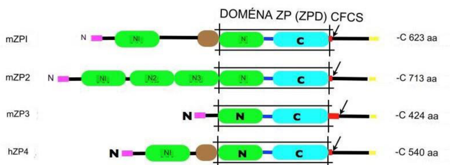
Obrázek 4. Znázornění organizace proteinů myši zony pellucidy (ZP) mZP1–3 a lidského ZP proteinu hZP4 (převzato a upraveno z Litscher & Wassarman 2020).
