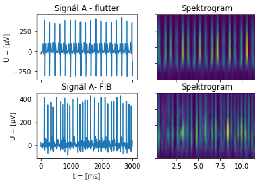
Obr. 6.4: Vytvořené spektrogramy
