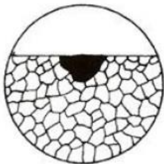
Obrázek 2: Důlková koroze [18]
