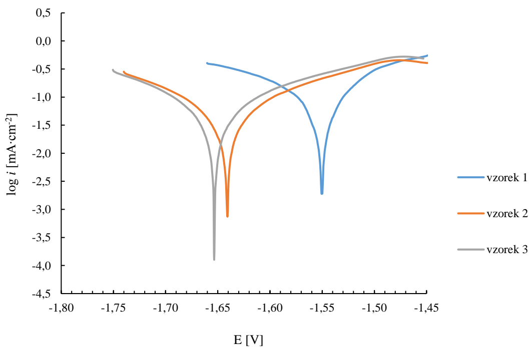
Obrázek 13: Polarizační křivky leštěných vzorků
