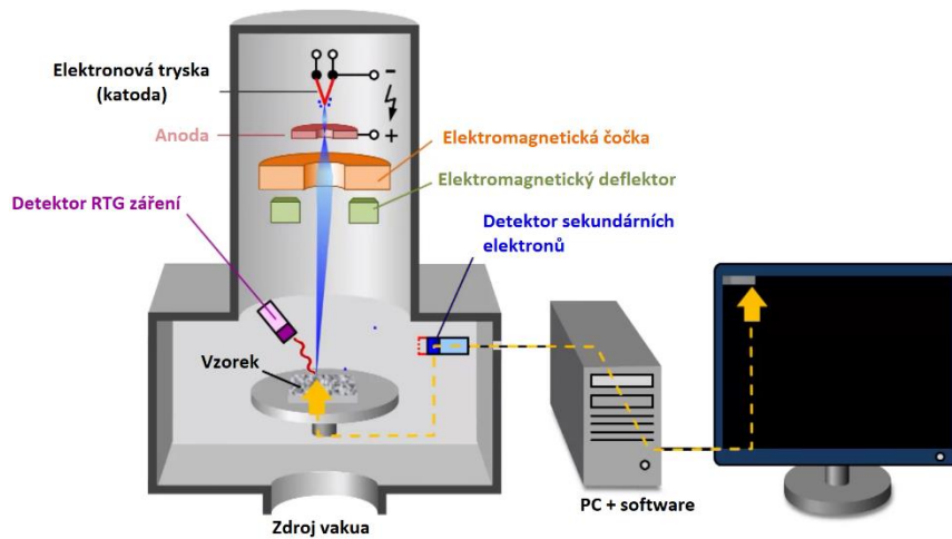
Obrázek 10: Schéma SEM [24]
