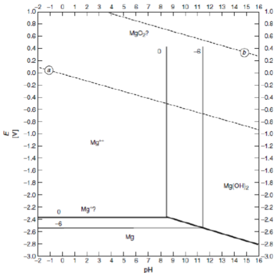
Obrázek 7: E-pH diagram hořčíku [19]
