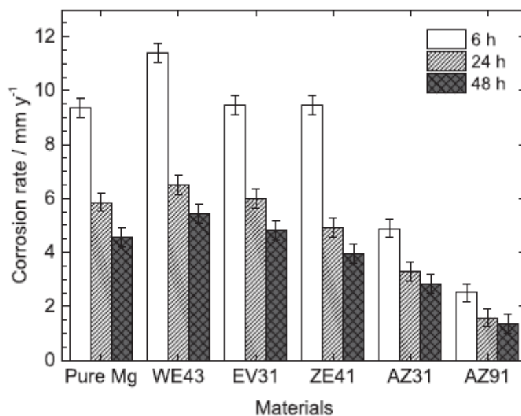
Obrázek 12: Porovnání korozních rychlostí vybraných hořčíkových slitin a čistého hořčíku po 6, 24 a 48 hodinách v 0,1 M Na 2 SO 4 [26]
