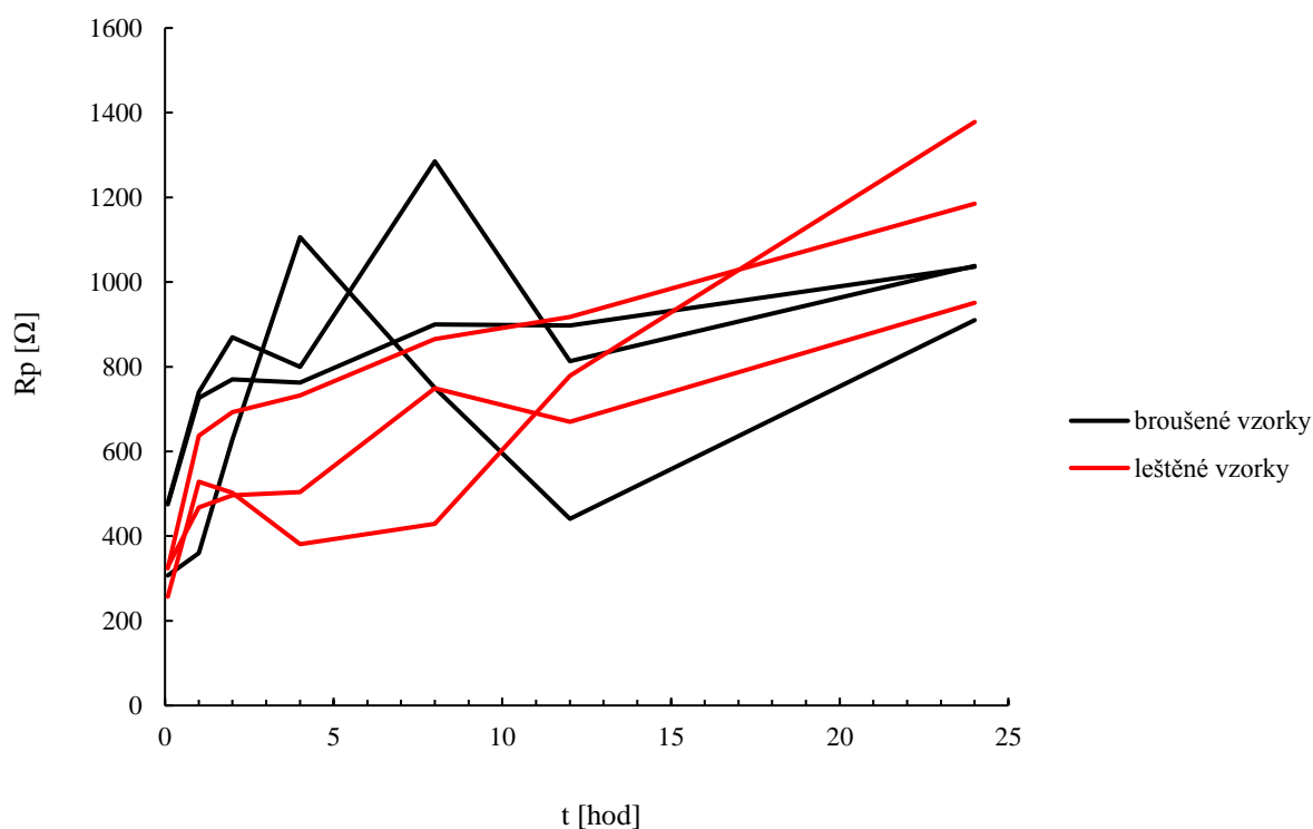
Obrázek 27: Časový vývoj polarizačního odporu, 5 min–24 hod
