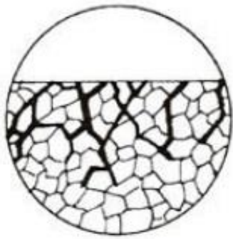
Obrázek 3: Mezikrystalová koroze [18]
