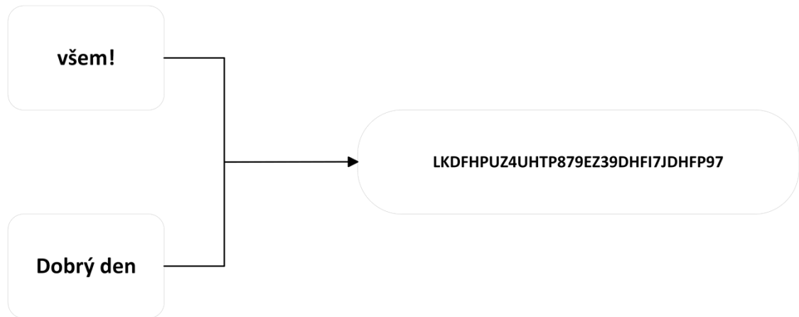
Obr. 2.5 Kombinované hashování
