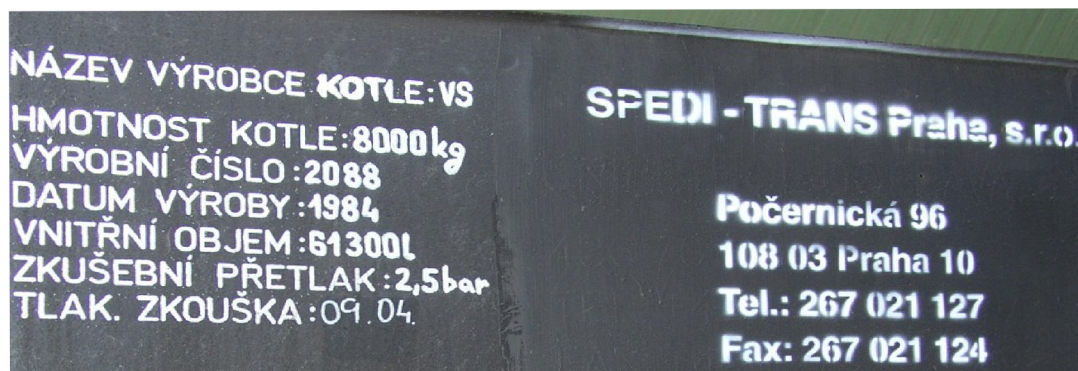
Obr. 2.6 Technické údaje a termín tlakové zkoušky
