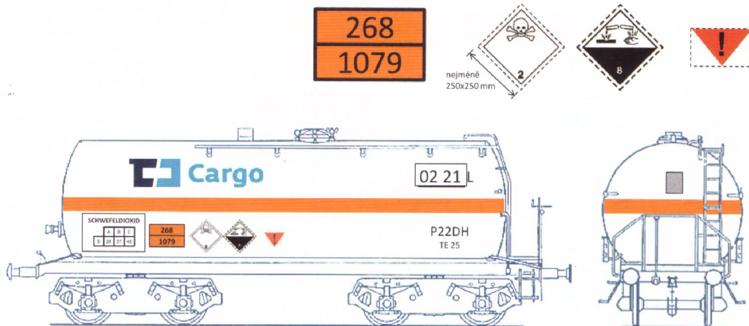
Obr. 1.2 Cisternový vůz s tabulkami a oranžovým pruhem
