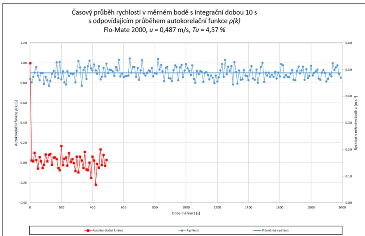
Graf 7.5 Časový průběh rychlosti za okrajové podmínky Cb včetně korelogramu pro Flo- Mate 2000
