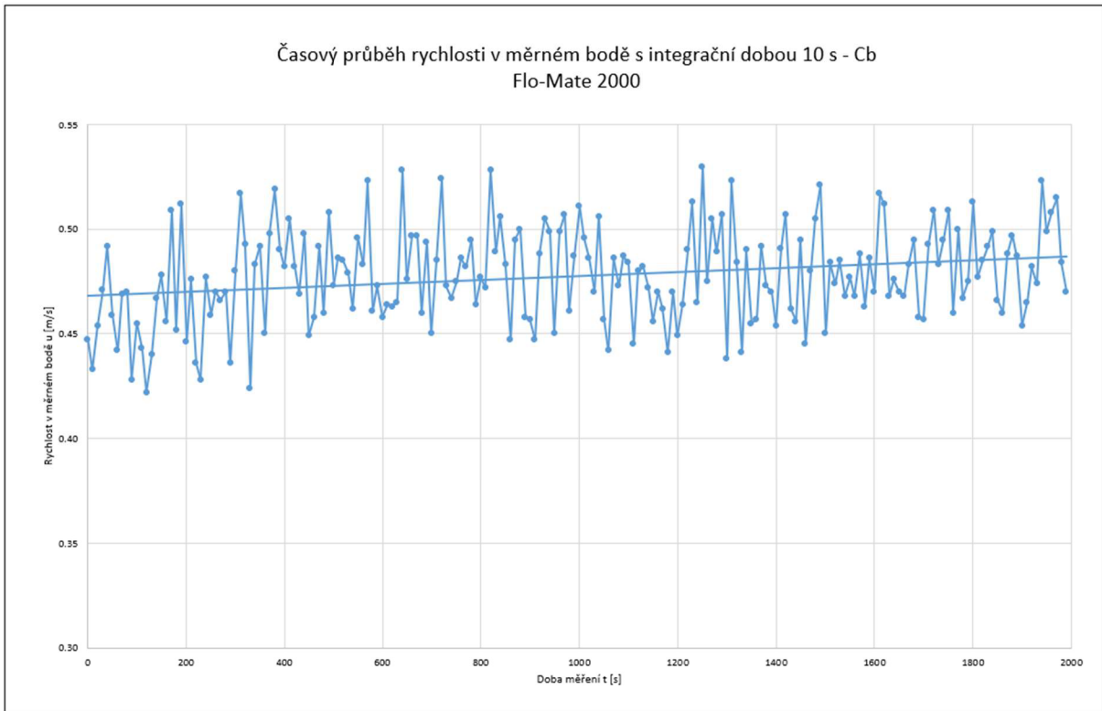
Graf 7.4 Časový průběh rychlosti při 2000 s trvajícím měření s Flo-Mate 2000 – okrajové podmínky Cb
