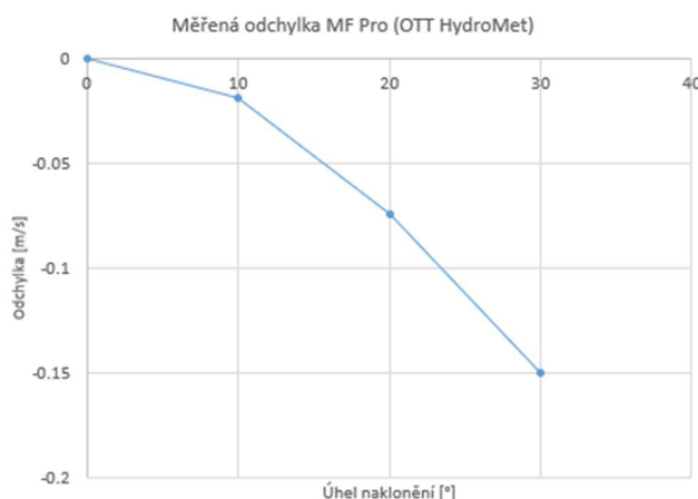
Graf 5.1 Závislost odchytky vykazované rychlosti na natočení snímače EMI měřidel MF Pro při rychlosti 0,61 m/s dle [9]
