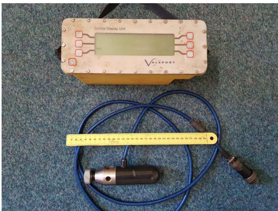
Obr. 7.3 EMI-měřidlo Valeport-Cylindrical model 801 s příslušenstvím
