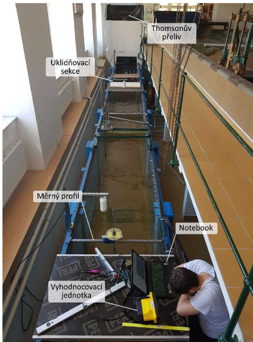
Obr. 7.1 Protiproudni pohled na měrný žlab
