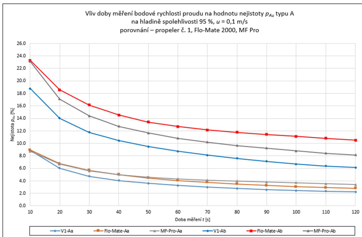
Graf 7.6 Nejistota ve stanovení bodové rychlosti pro všechna posuzovaná měřidla při u = 0,1 m/s
