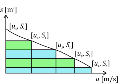
Obr. 3.7 Stanovení průtoku
