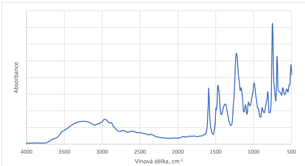
Graf 3: FTIR spektrum vlastní syntetizované lignin-fenol-formaldehydové pryskyřice
