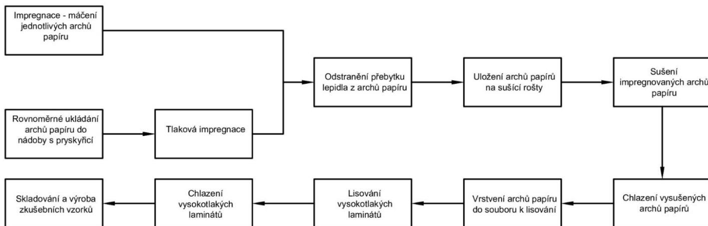
Obrázek 14: Schéma laboratorní výroby vysokotlakých laminátů (Vlastní zpracování)
