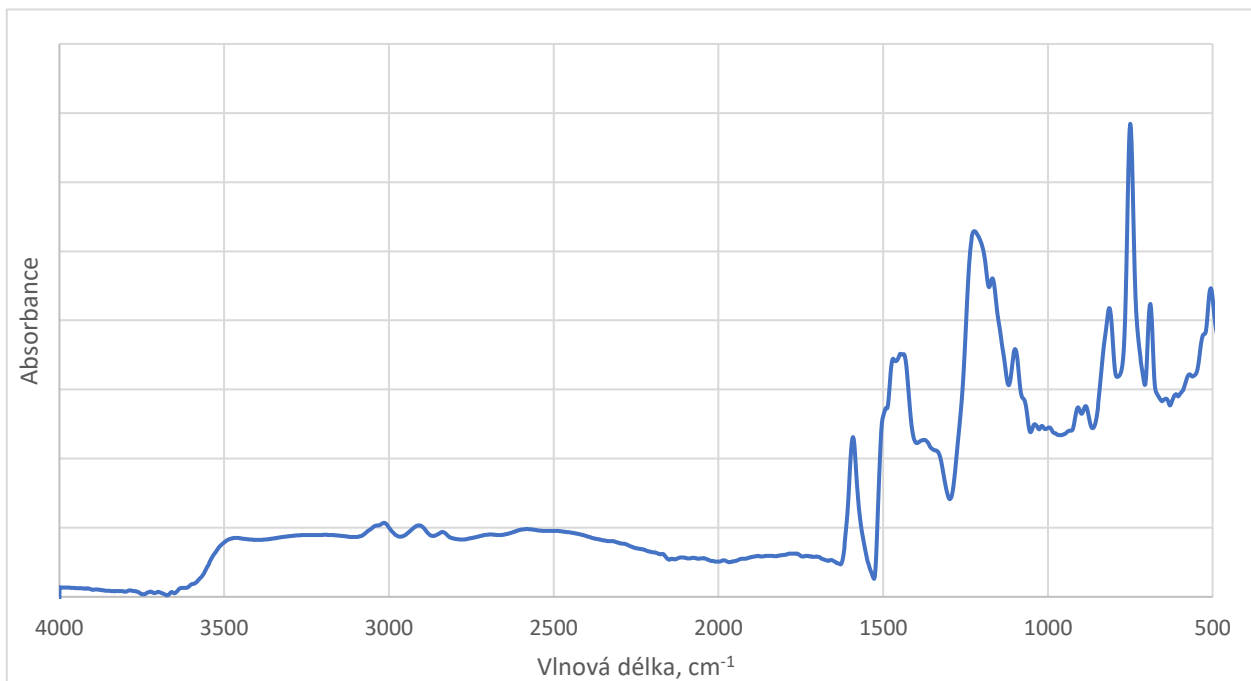
Graf 4: FTIR spektrum vytvrzené vlastní syntetizované lignin-fenol-formaldehydové pryskyřice
