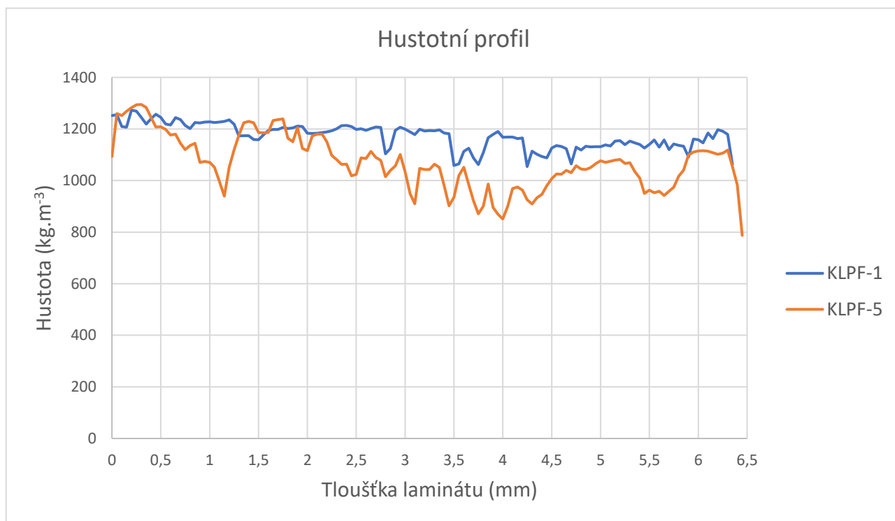
Graf 17: Hustotní profil laminátů KLPF-1 a KLPF-5
