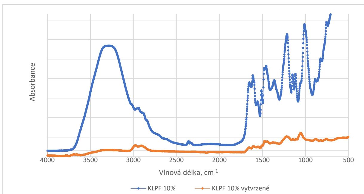
Graf 7: FTIR spektrum komerční PF pryskyřice s přidavkem ligninu 10 % (KLPF-10)
