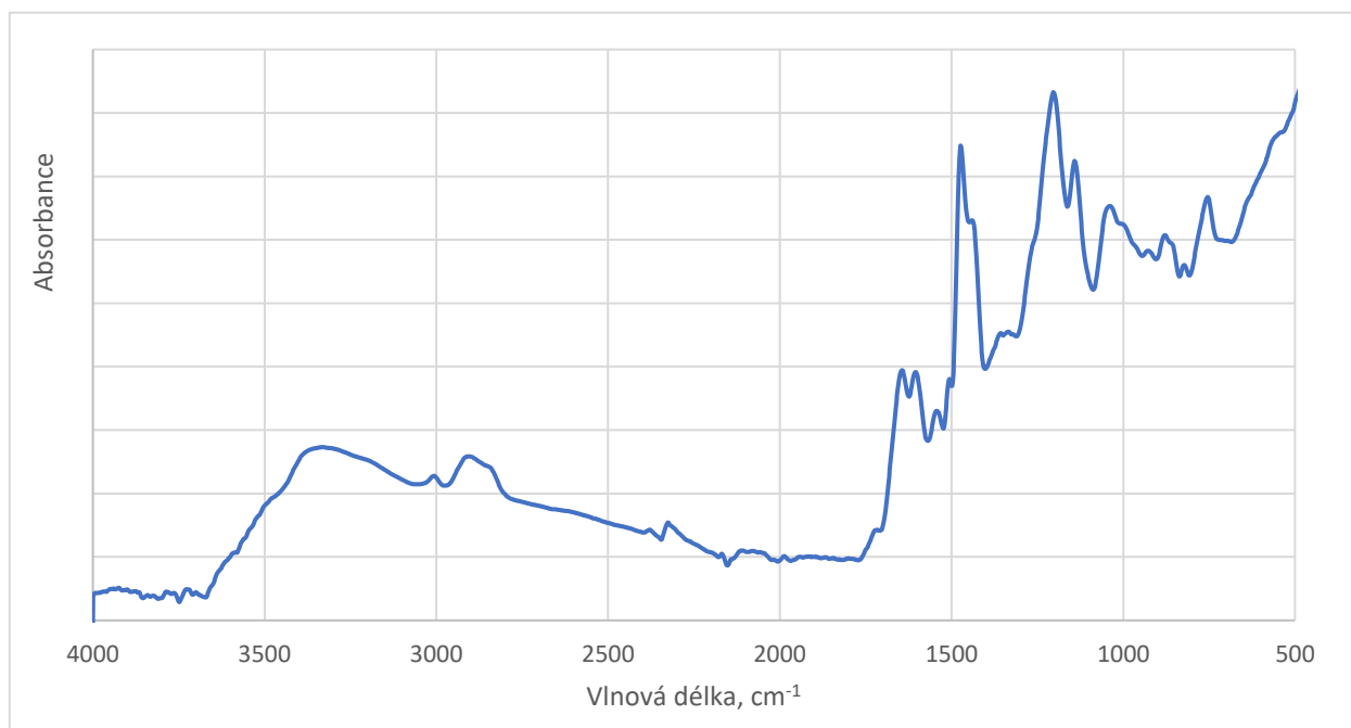
Graf 2: FTIR spektrum vytvrzené fenol-formaldehydové pryskyřice
