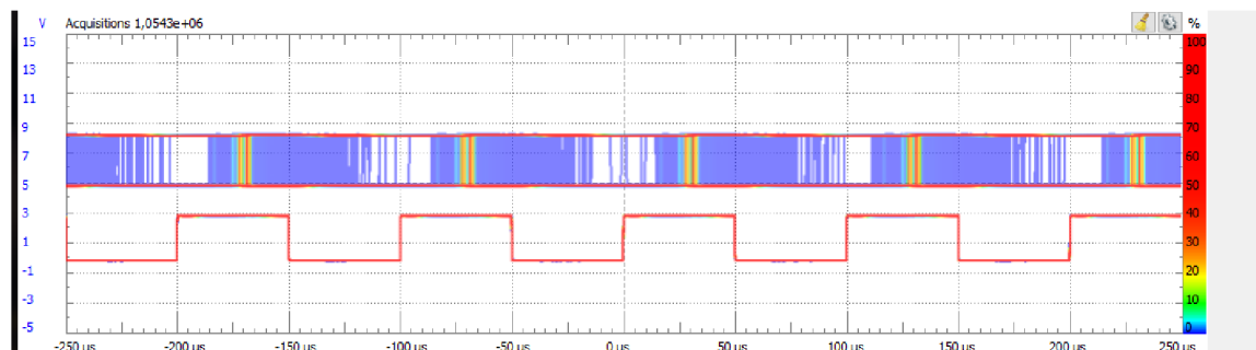
Obrázek 8.2.1 Výsledek měření latence na základě vyvolání přerušení pro plánovací politiku typu FIFO bez zatíženého systému
