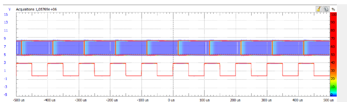
Obrázek 8.2.3 Výsledek měření latence na základě vyvolání přerušení pro plánovací politiku typu RR se zatěží systému
