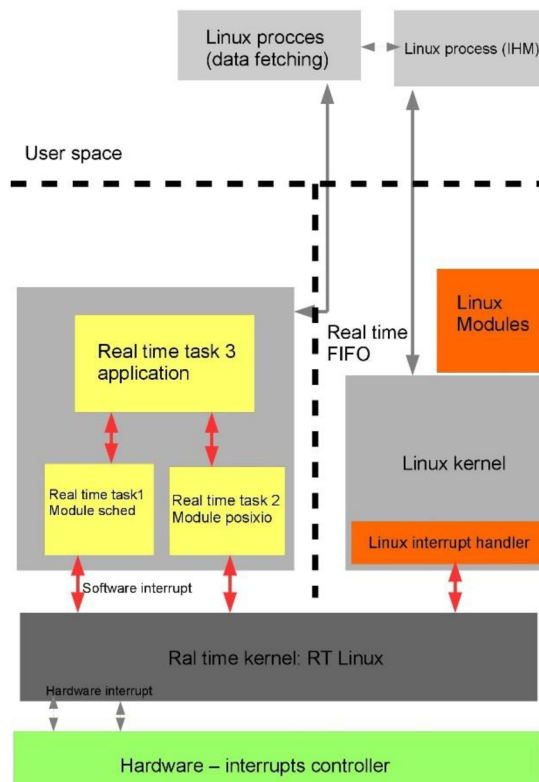
Obrázek 2.1.3 RTLinux architektura [4]
