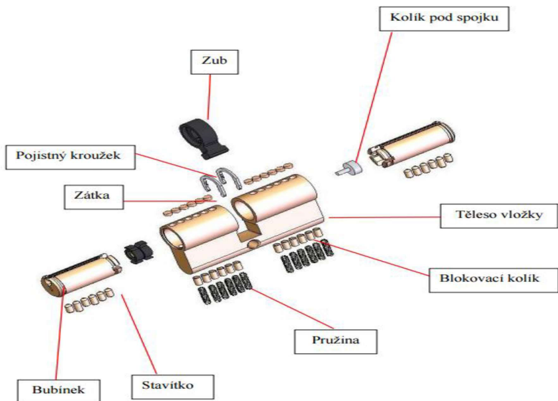
Obr. č. 8: Popis oboustranné cylindrické vložky. Zdroj: (autor práce).
