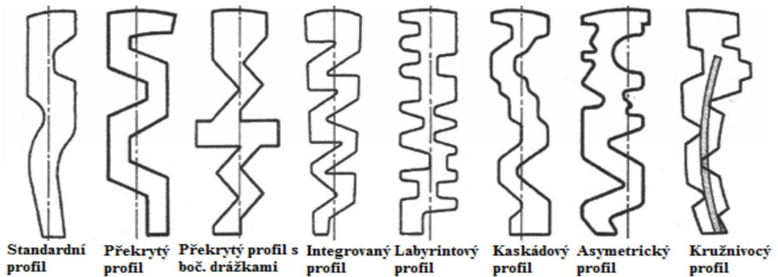
Obr. č. 10: Profily klíče. Zdroj: (UHLÁŘ, J. Technická ochrana objektů I. díl: Mechanické zábranné systémy II . Praha: Vydavatelství PA ČR, 2004. s. 94. ISBN 978-80-7251-312-3).
