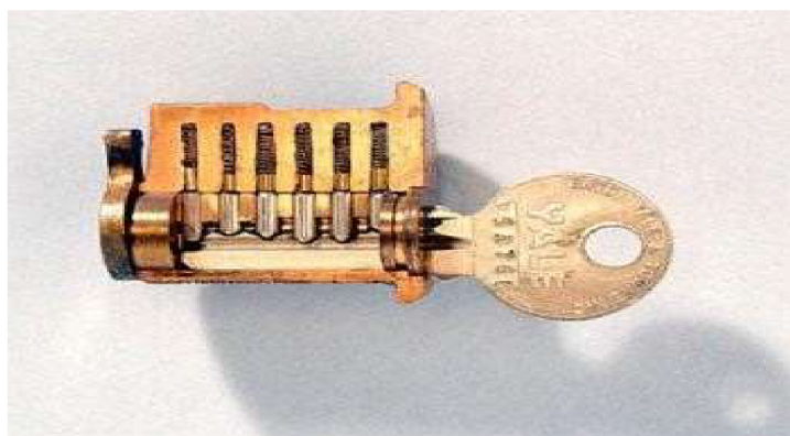
Obr. č. 3: Cylindrická vložka Linuse Yalea. Zdroj: ( http://www.zapaservis.com/Historie%20zamku.pps ).
