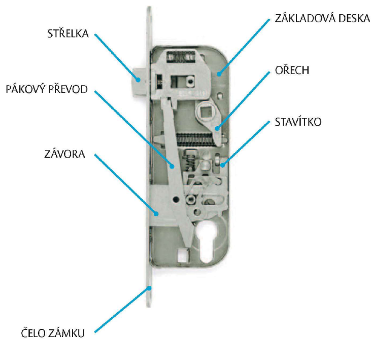
Obr. č. 7: Zadlabací zámek. Zdroj: (autor práce).
