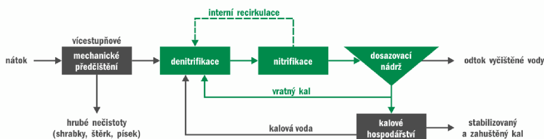
Obrázek 1 Zjednodušené technologické schéma ČOV[2]
