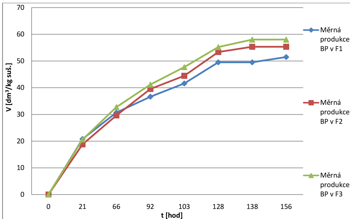
Graf 3 Měrná produkce bioplynu při třetím experimentu
