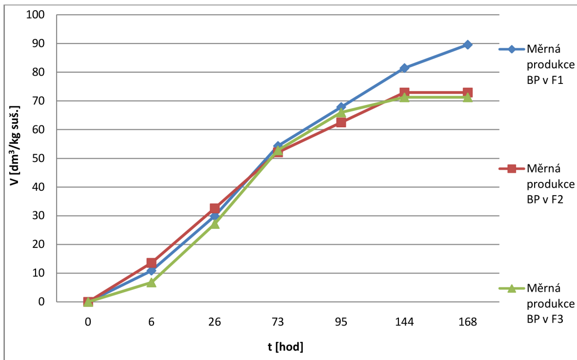
Graf 1 Měrná produkce bioplynu při prvním experimentu
