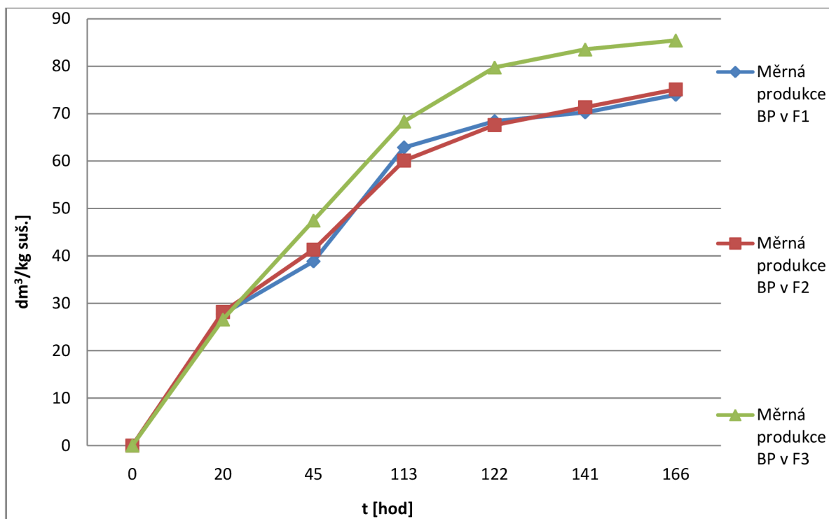
Graf 2 Měrná produkce bioplynu při druhém experimentu
