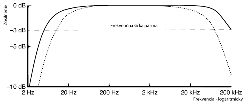
Obr. 1.1: Frekvenčný rozsah audio zosilňovača [1].
