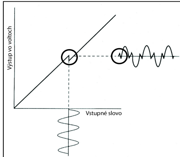
Obr. 1.8: Chyba pri prevode malých signálov so znamienkom [11].
