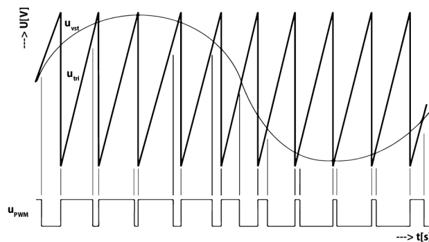
Obr. 1.4: Priebehy vstupných a výstupných signálov komparátora v triede D [3].
