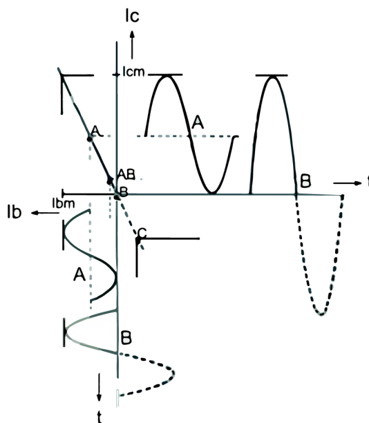
Obr. 1.3: Pracovné triedy zosilňovačov [9].
