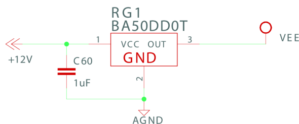
Obr. 3.13: Schéma zapojenia regulátora BA50DD0T pre napájanie Raspberry Pi.
