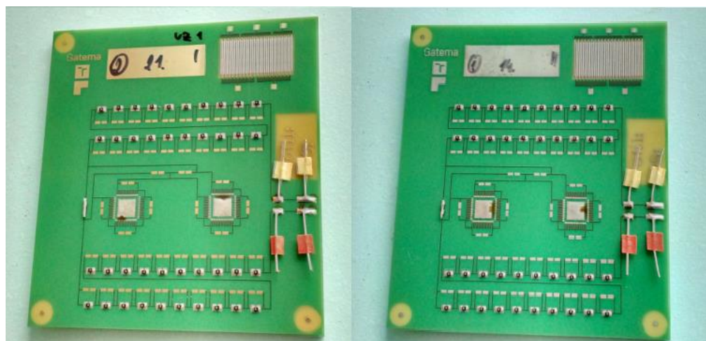
Obrázek 18: Měřené vzorky s povrchovou úpravou ENIG a imerzní cín
