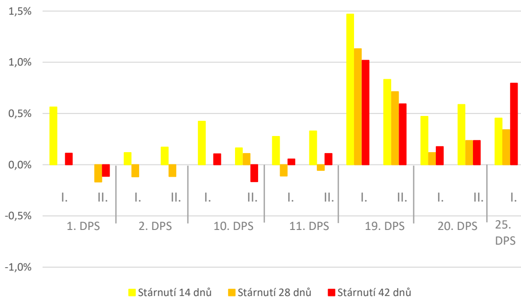
Graf 18: Procentuální změna odporu po 42 dnech stárnutí v mrazicím boxu, povrchová úprava imerzní cín
