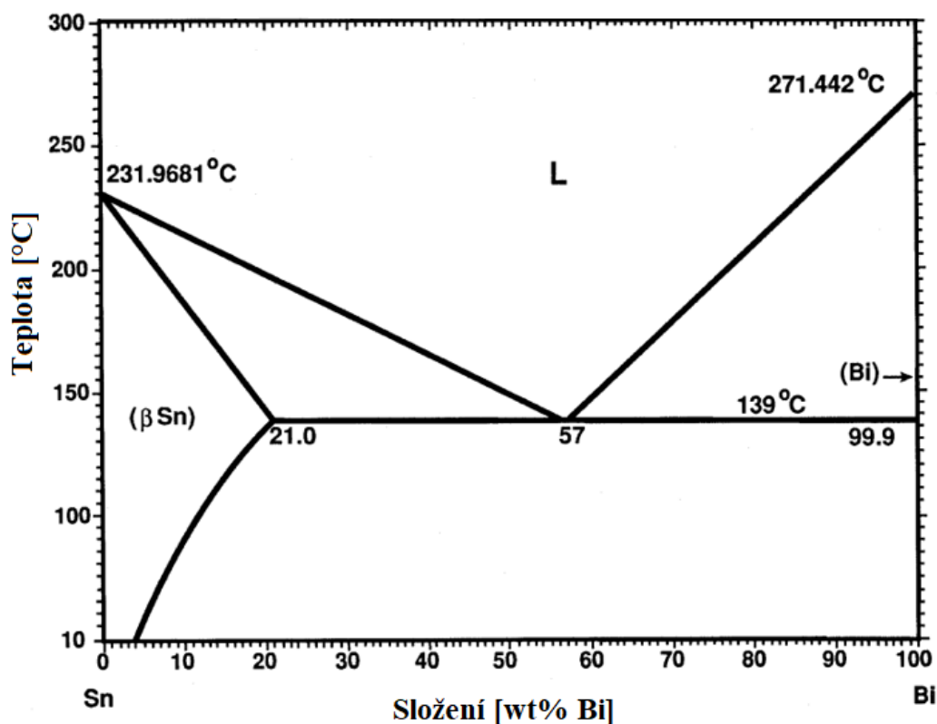
Obrázek 2: SnBi fázový diagram (převzato z [5])
