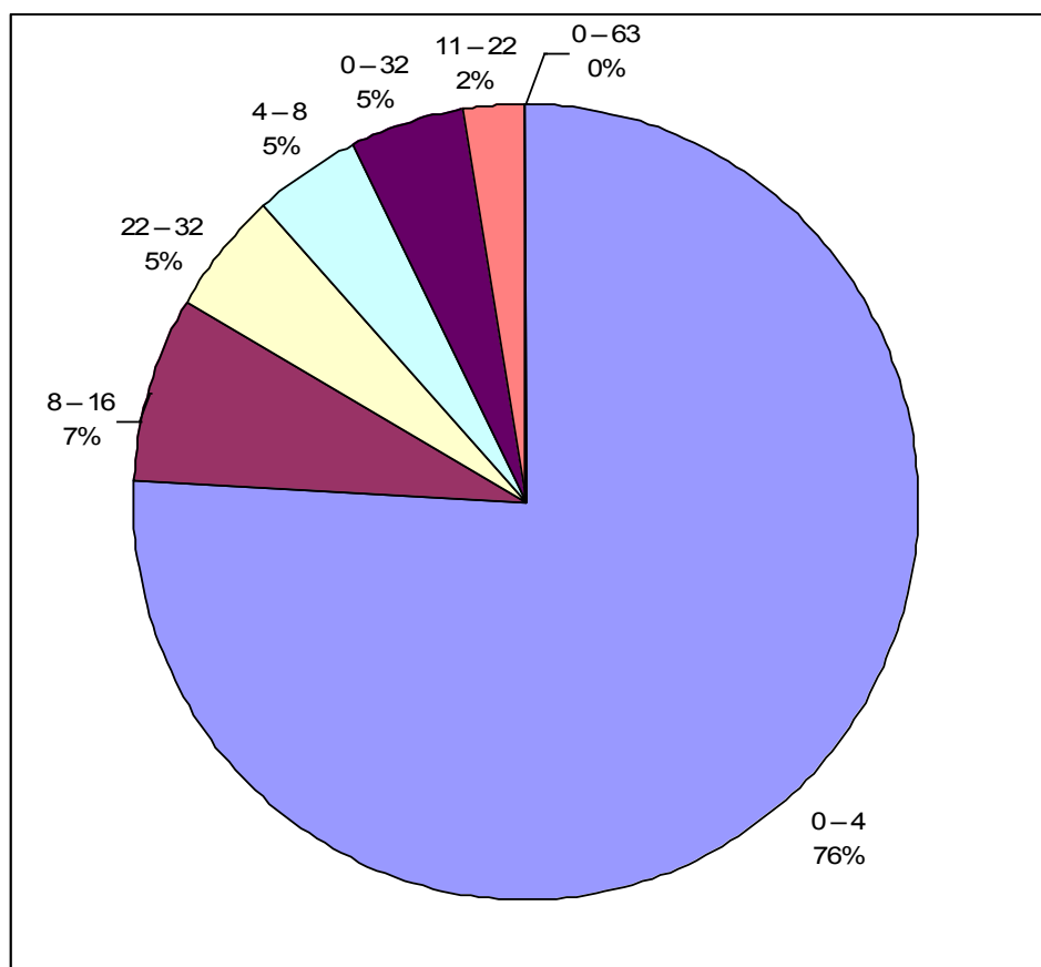
Obr. 8.1.2.: Frakční složení (v %) expedice pískoven Písková Lhota a Vrbová Lhota za rok 2009, zdroj: Pískovny Hrádek, a. s. (2010), vlastní úprava
