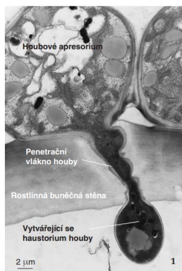
Obrázek 8: Apresorium houby Magnaporthe oryzae pronikající přes buněčnou stěnu do rostlinné buňky (převzato ze: Sabol a Pilátová 2020).
