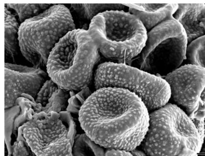
Obrázek 18: Spory S. destruens zobrazeny skenovací elektronovou mikroskopií (SEM) (převzato z: https://www.padil.gov.au/ ).
