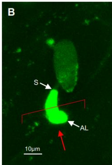
Obrázek 13: Detekce NO v apresoriu klíčící konidie padlí Blumeria graminis f. sp. hordei pomocí DAF-2 DA (převzato z: Prats et al. 2008).
