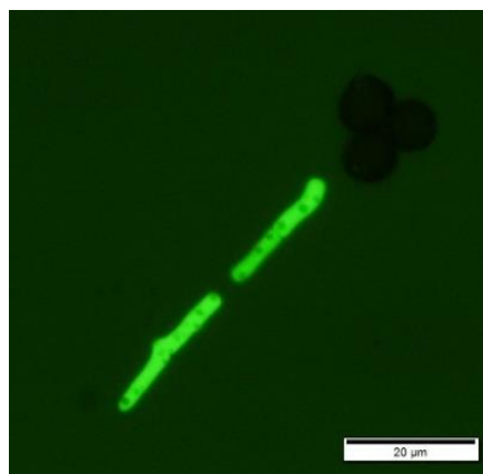
Obrázek 34: Detail tří spor S. destruens , z nichž pouze jedna klíčí vláknem vykazujícím signály ROS – zelená fluorescenci (inkubace 4 dny v pokojové teplotě (~ 22 °C), barvení pomocí H 2 DCF-DA). Autor: A. Bobková.
