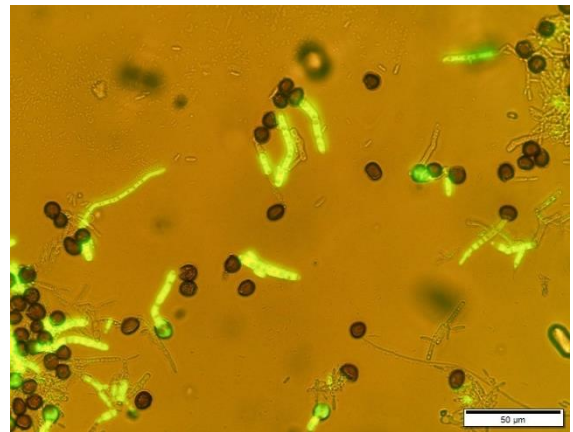
Obrázek 33: Shluky klíčících spor S. destruens se signálem ROS v klíčcích vlákněch vykazujícím fluorescenci (inkubace 4 dny při teplotě 20/17 °C (12/12 h), barvení pomocí H 2 DCF-DA). Autor: A. Bobková.
