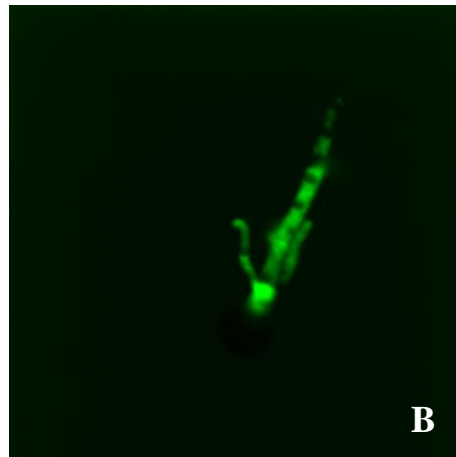
Obrázek 44: Spora S. destruens s rozvětveným klíčným vláknem (inkubace 5 dní při teplotě 15/10 °C (12/12 h), barvení pomocí DAF-FM DA). A – snímek pořízen kombinací kanálů, Nomarského diferenciální kontrast a fluorescence, B – pouze fluorescence DAF-FM DA. Autor: A. Bobková.
