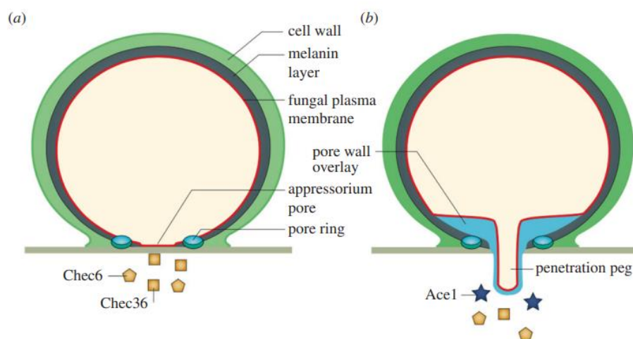
Obrázek 7: Znárodnění procesu pronikání vláknitých hub do rostlinného pletiva. (a) přichycení apresoria k povrchu listu (b) osmotický tak vtačuje penetrační hrot houby do rostlinného pletiva (převzato ze: Segal 2016).
