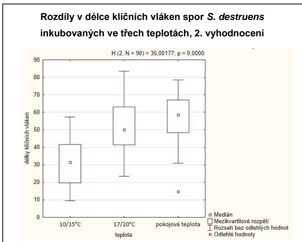
Obrázek 29: Rozdíly v délce klíčnicích vláken (v \mu\text{m} ) spor S. destruens inkubovaných ve fytotronu v teplotě 15/10 °C (12/12 h světlo/tma), 20/17 °C (12/12 h světlo/tma) a v laboratoři v pokojové teplotě (9/15 h světlo/tma). Porovnávány hodnoty z 2. vyhodnocení.
