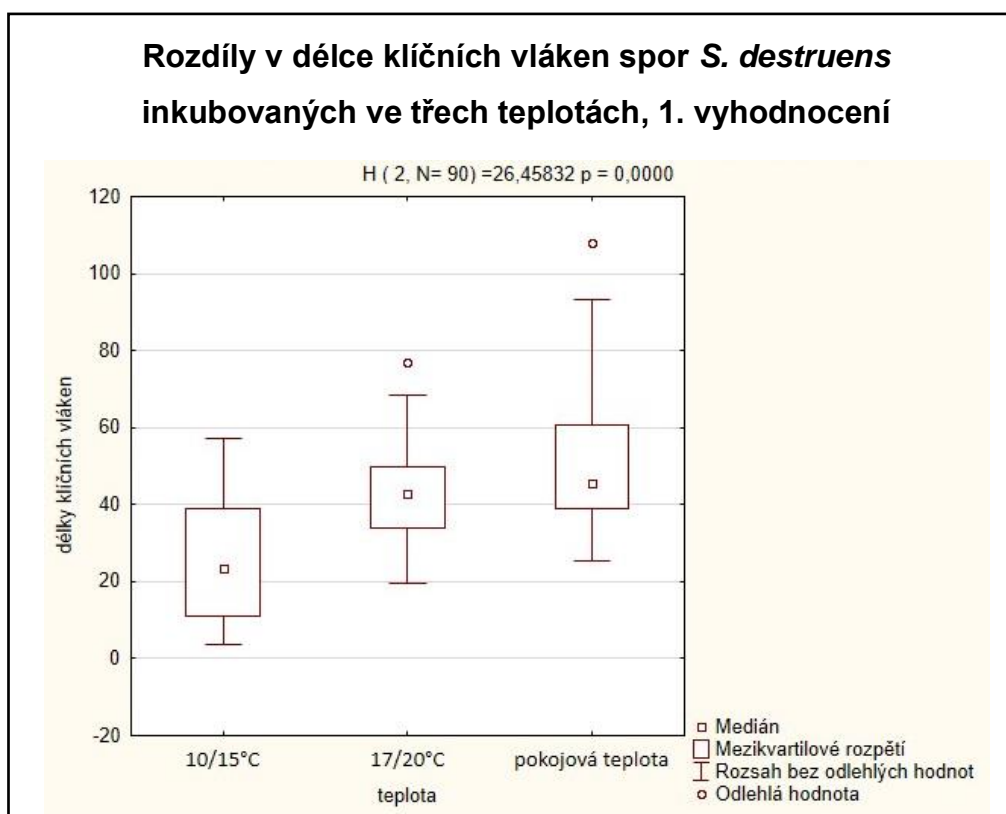
Obrázek 28: Rozdíly v délce klíčních vláken (v \mu\text{m} ) spor S. destruens inkubovaných ve fytotronu v teplotě 15/10 °C (12/12 h světlo/tma), 20/17 °C (12/12 h světlo/tma) a v laboratoři v pokojové teplotě (9/15 h světlo/tma). Porovnávány hodnoty z 1. vyhodnocení.
