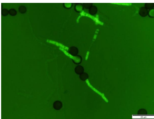
Obrázek 23: Mikrofotografie klíčících spor S. destruens v různém stádiu klíčení (7 dní). V některých případech je viditelná fluorescence i ve sporách (začátek klíčení), v jiných pouze v klíčícím vlákně, v dalších případech fluorescence z klíčících vláken pomalu mizí (pokročilejší fáze klíčení). Autor: A. Bobková.
