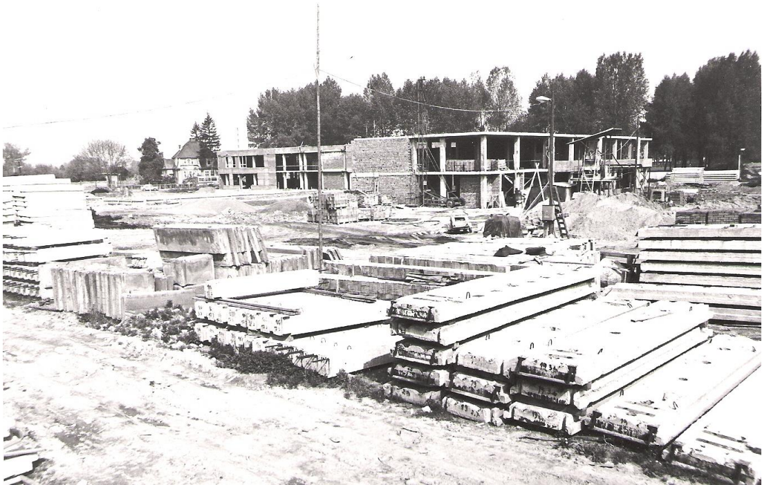
Obrázek 17 Hrubá stavba ZDŠ U Stadionu
