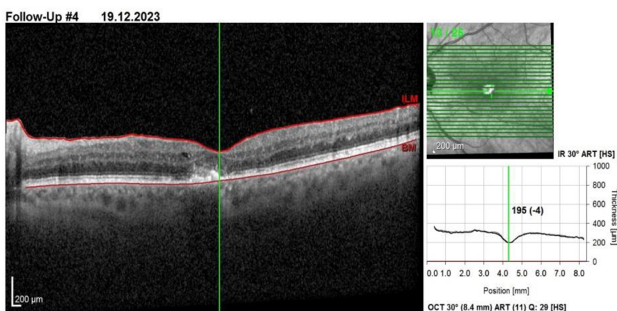
Obr. 22 - OCT sítnice
