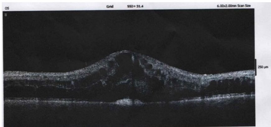
Obr. 14 - OCT sítnice
