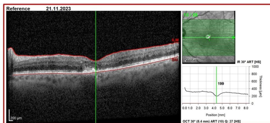
Obr. 21 - OCT sítnice
