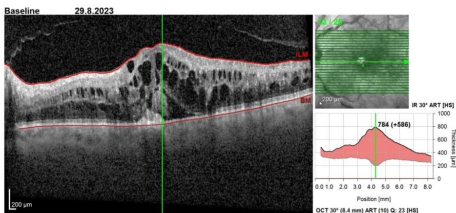
Obr. 15 - OCT sítnice
