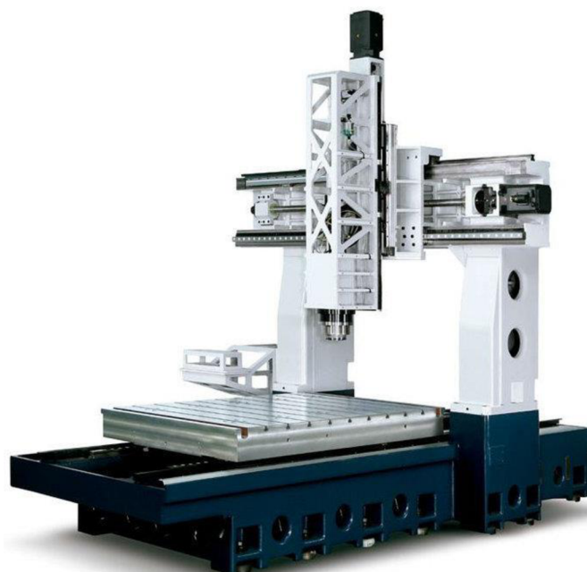
obr. 2.3 Vertikální obráběcí centrum [38]
