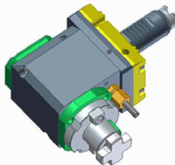
obr. 3.7 Pravoúhlá frézovací hlava [13]
