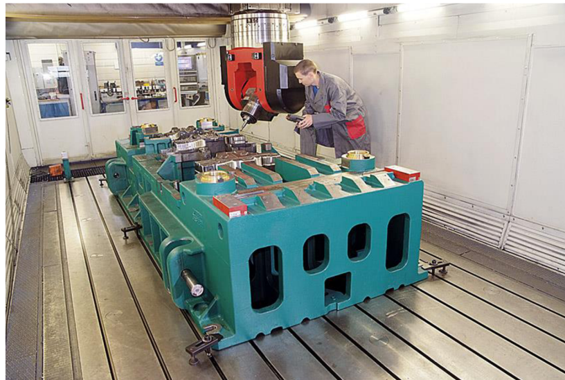
obr. 4.2 Vnitřní část stroje TRIMILL 6525 [41]
