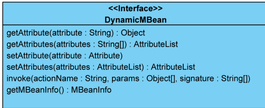
Obrázek 6.2: Definice rozhraní DynamicMBean
