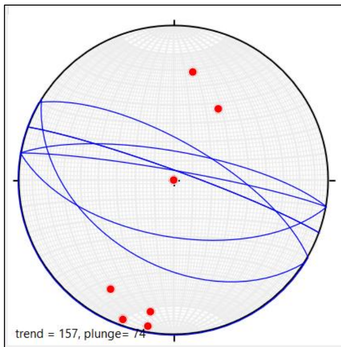
Obrázek 20 - Tektonogram puklin u první lokality (Stereonet)
