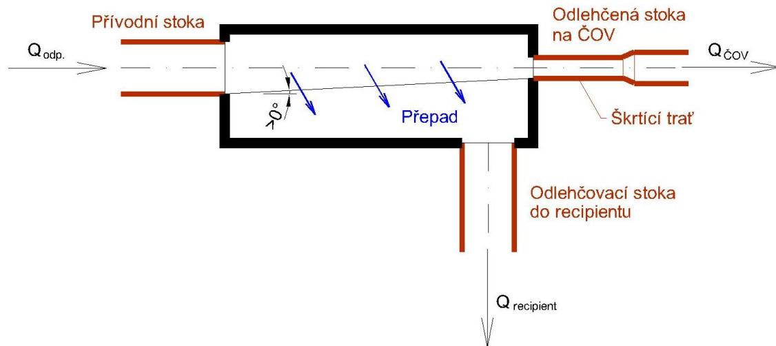
Obr. 3.10. OK s přepadem bočním se šikmou hranou a se škrťací trať
