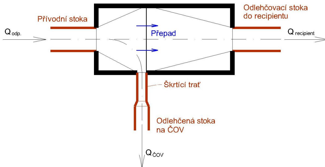
Obr. 3.9. OK s přepadem přímým kolmým se škrťací tratí
