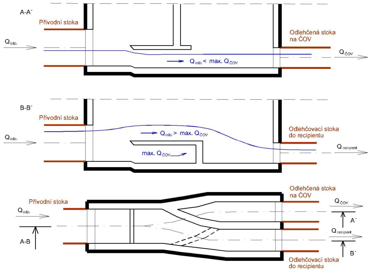
Obr. 3.12. OK s horizontální dělicí stěnou
