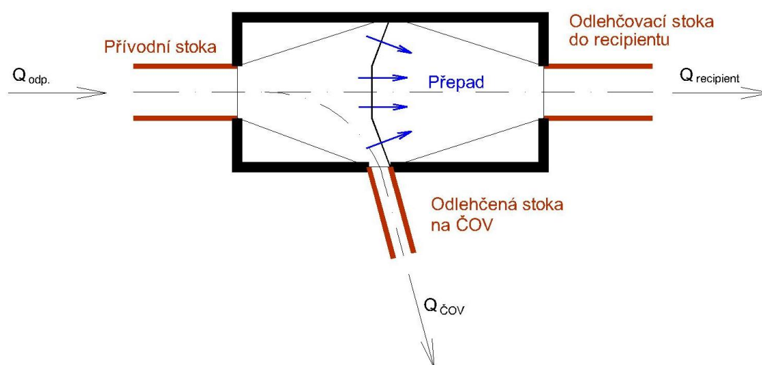
Obr. 3.4. OK s přepadem přímým lomeným
