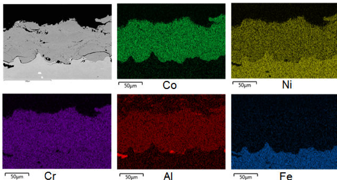
Obr. 4.10 Výsledky mapování chemického složení vzorku HV0
