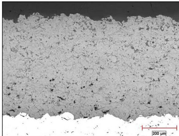
Obr. 2.3 Mikrostruktura svrchního keramického povlaku naneseného plasmovým nástřikem [2]
