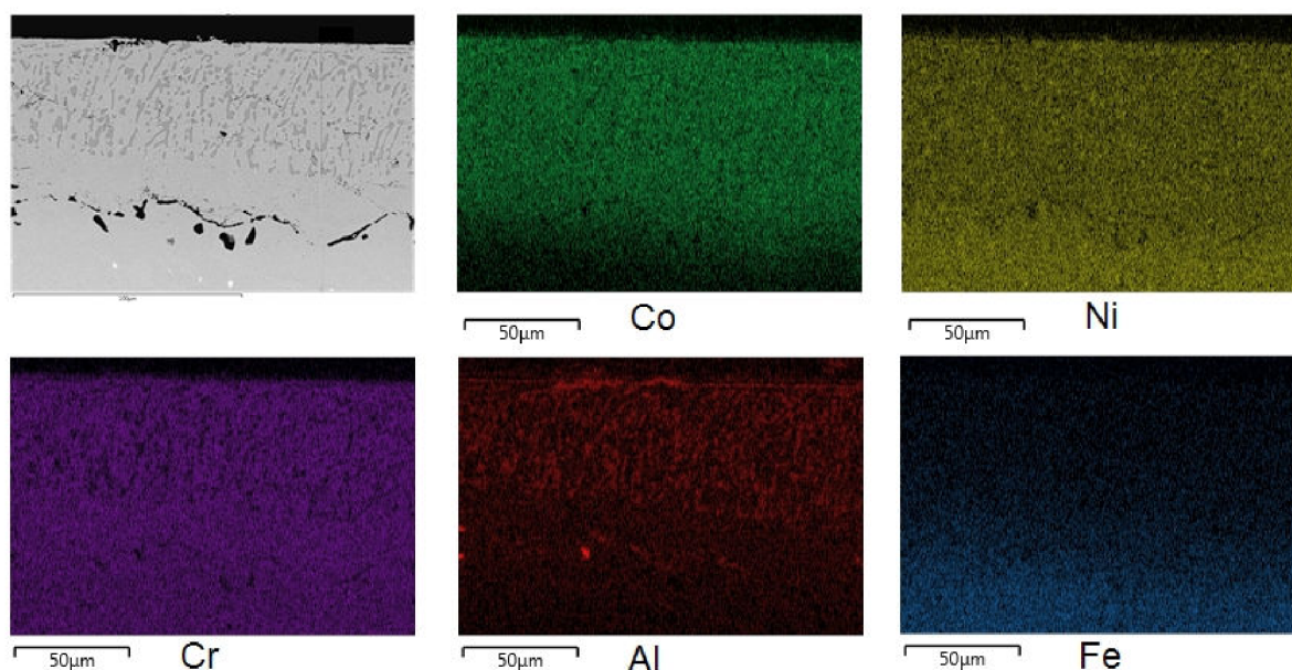
Obr. 4.42 Mapování chemického složení vzorku HV4HT
