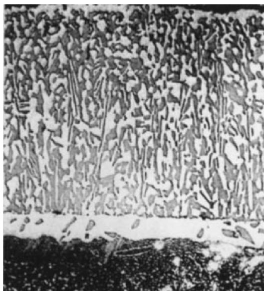
Obr. 2.2 Mikrostruktura \text{MCrAlY} vazebného povlaku [3], kde světle šedá je matrice tvořená tuhým roztokem \gamma a tmavě šedá je fáze \beta\text{-NiAl}
