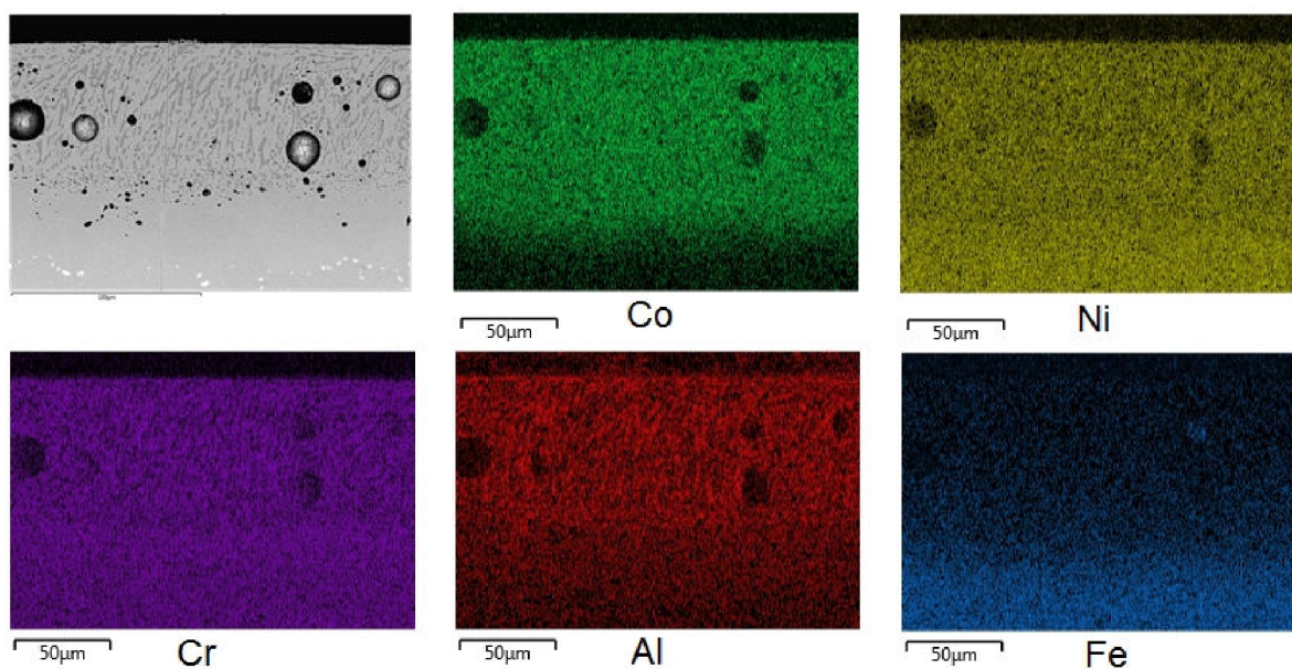
Obr. 4.41 Mapování chemického složení vzorku CS4HT
