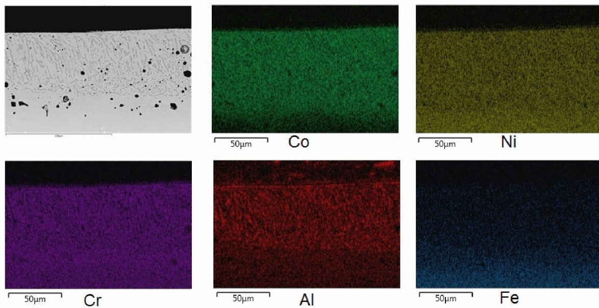
Obr. 4.36 Mapování chemického složení vzorku CS2HT
