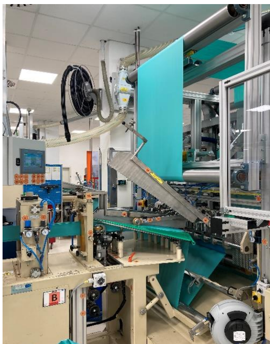
Obrázek 10 Foto modulu kladek (vlastní zpracování)
