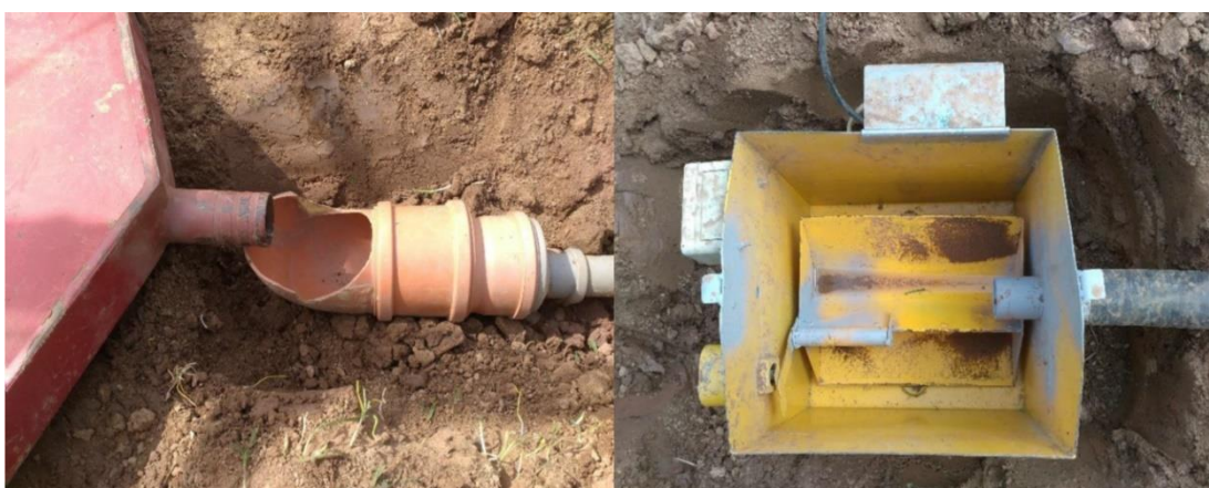
Obrázek č. 22: Člunkový průtokoměr vlevo a překlápečka vpravo (VÚMOP, 2018).
