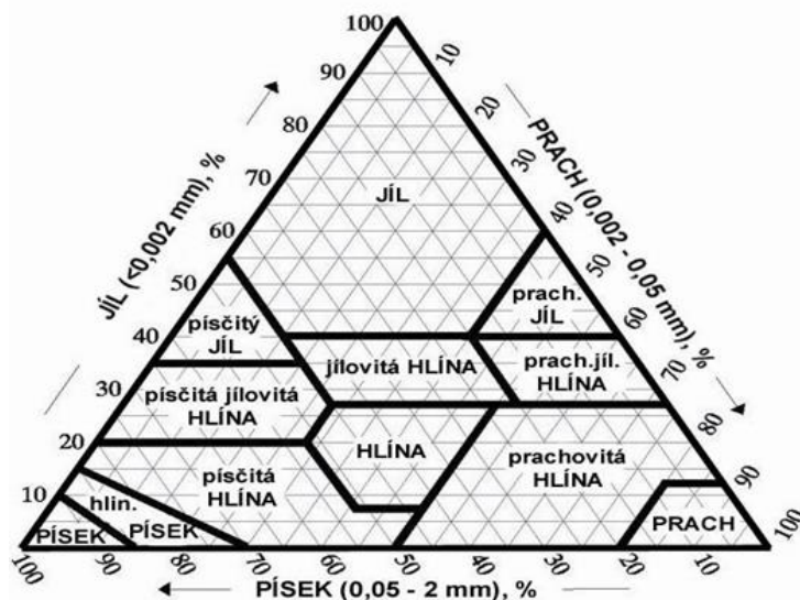
Obrázek č. 4: Trojúhelníkový diagram zrnitosti půd (Němeček a kol., 2001).
