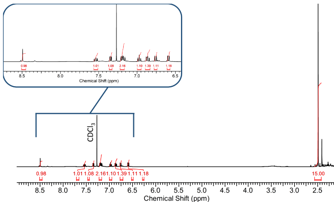
Obrázek č. 29: 1 H NMR spektrum komplexu [Ta(η 5 -Cp*)(OTF) 2 (salaph)] ( 7 ); vzorek byl připraven rozpuštěním v CDCl 3
