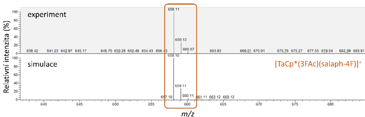
Obrázek č. 24: Porovnání ESI + hmotnostního spektra komplexu [Ta( \eta^5 -Cp*)(DCA) 2 (salaph-4F)] + (4) (nahore) a simulace izotopového rozložení pro iont [M-(DCA)] + (dole).
