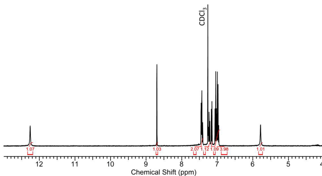
Obrázek č. 26: ^1\text{H} NMR spektrum 2- \{(E)-[(2\text{-hydroxyfenyl)imino]methyl}\} fenolu ( \text{H}_2\text{salaph} ); vzorek byl připraven rozpuštěním v \text{CDCl}_3
