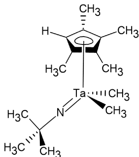
Obrázek č. 9: Strukturální vzorec komplexu (\eta^5\text{-C}_5\text{Me}_4\text{H})\text{Ta}(\text{=N}^t\text{Bu})\text{Me}_2 [40]
