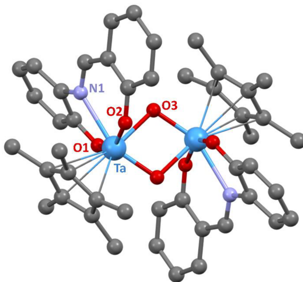
Obrázek č. 33. Molekulová struktura dvojjaderného komplexů [\text{Ta}(\mu\text{-O})(\eta^5\text{-Cp}^*)(\text{salaph})_2] ( 8 ). Vodíkové atomy byly pro přehlednost vynechány.
