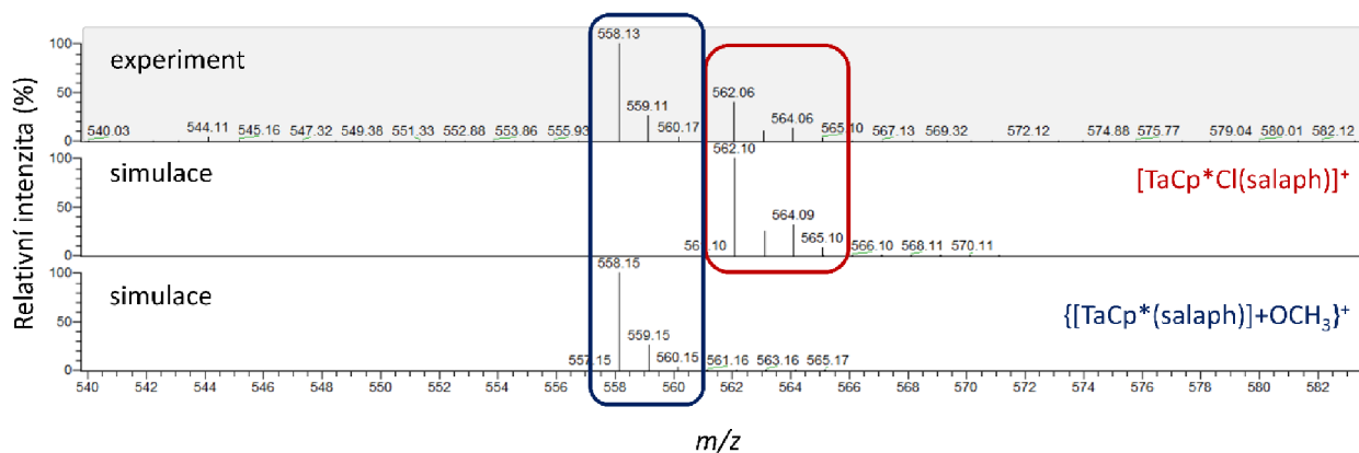
Obrázek č. 23: Porovnání ESI + hmotnostního spektra komplexu [TaCp*Cl(salaph)] + (1) (nahore) a simulace izotopového rozložení pro ionty [M-Cl] + (uprostřed) a methanoláto aduktu o složení {(M-2Cl)+OCH 3 } + .
