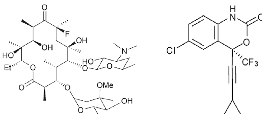
Obrázek č. 21: Struktura Flurithromycinu a Efavirenz
