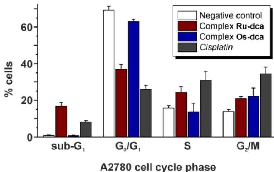
Obrázek č. 16: Srovnání procentuálního počtu buněk nádoru typu A2780 po aplikaci cisplatinu, komplexu Ru-DCA, komplexu Os-DCA vůči negativní kontrole v jednotlivých fázích buněčného cyklu po inkubační době 24 hodin
