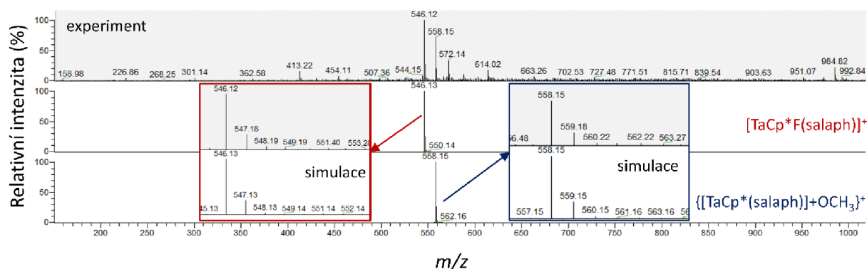
Obrázek č. 37: Porovnání ESI + hmotnostního spektra produktu syntézy fluoro komplexu (nahore) a simulace izotopového rozložení pro ionty [\text{M-F}]^+ (uprostřed) a methanoláto aduktu o složení \{[\text{TaCp}^*(\text{salaph})]+\text{OCH}_3\}^+ .
