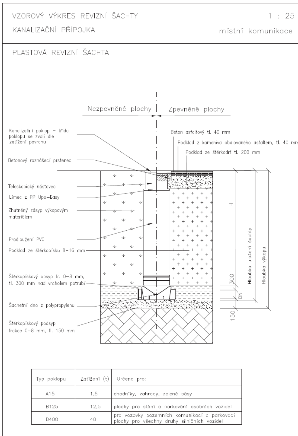
Obr. 4.4 Ukázka výkresu revizní šachty
