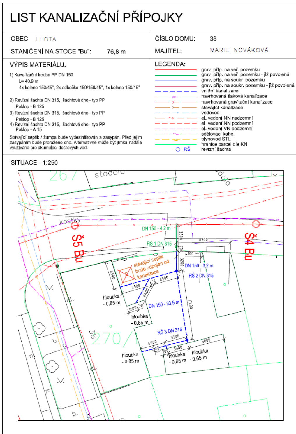
Obr. 4.5 Ukázka situace nemovitosti s půdorysem přípojky
