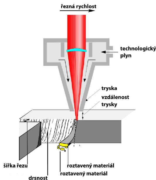
Obr. 41 Princip řezání laserem [36]
