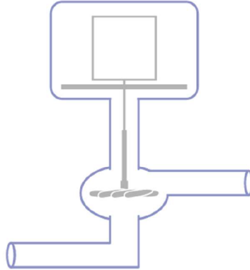
Obr. 7: Schéma bezucpávkového čerpadla [39]
