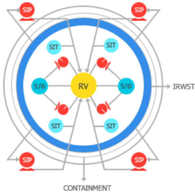
Obr. 14: Schéma bezpečnostního vstřikovacího systému reaktoru APRI400 [61]
