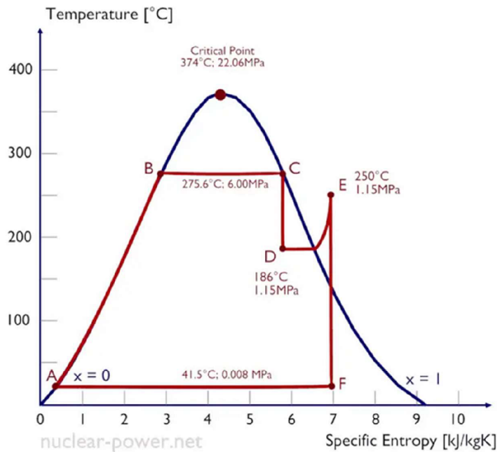
Obr. 2: Rankineův-Clausiov cyklus PWR reaktoru [6]
