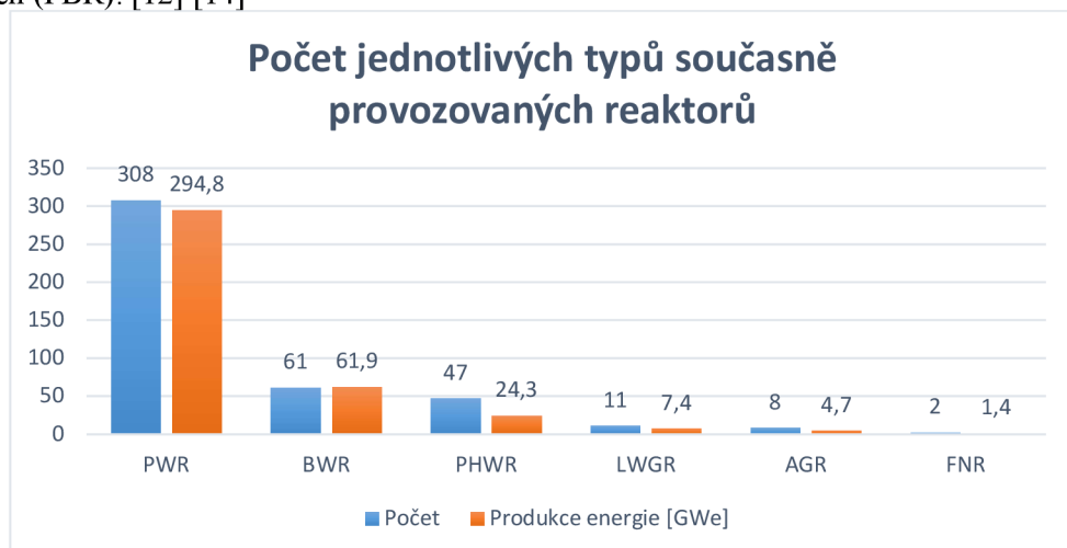
Obr. 5: Graf využití jednotlivých typů reaktorů v současnosti [12]
