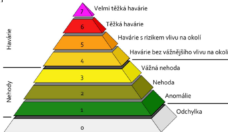
Obr. 9: Stupnice INES [42]
