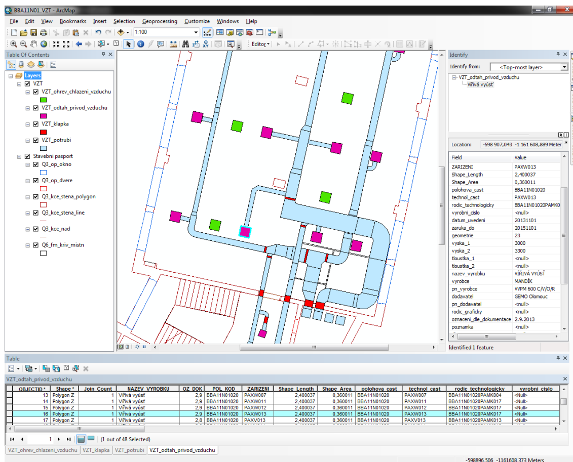
Obrázek 6-1 - Technologie VZT v patře N01 budovy BBA11
