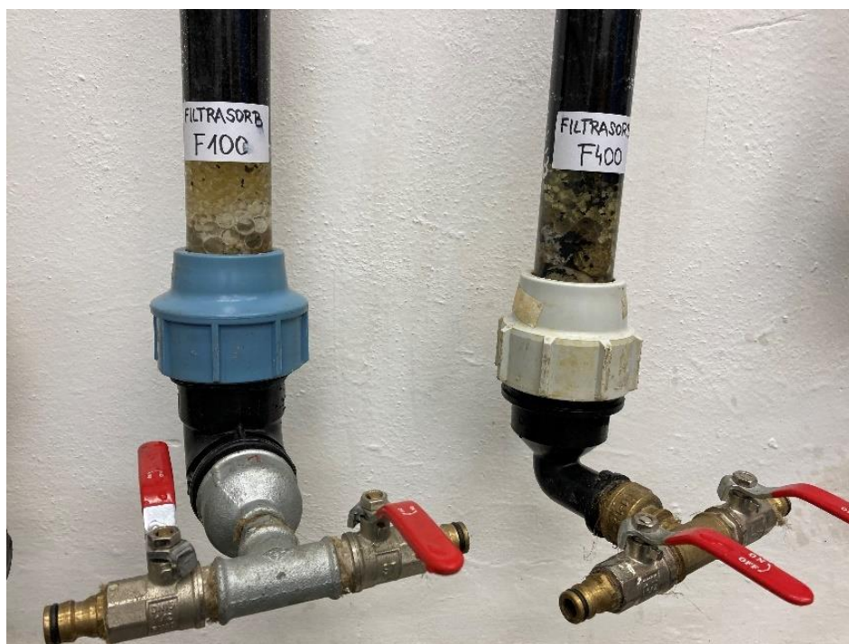
Obr. 47 Odběrné uzávěry kolon s přichystanými adsorbenty [autor]
