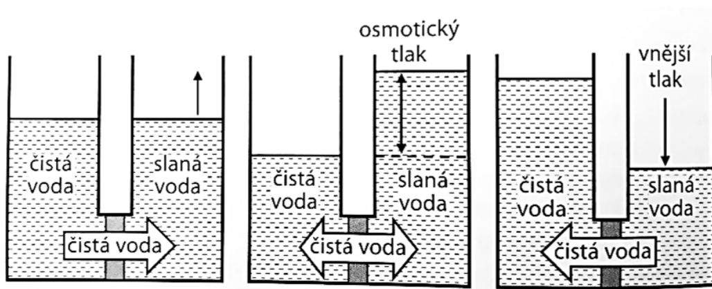
Obr. 4 Princip osmózy a reverzní osmózy [18]
