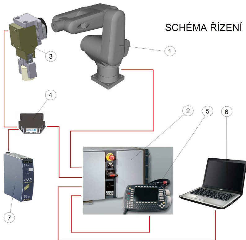
Obr. 9-14.: Schéma řízení [32], [53], [80], [81], [82]
