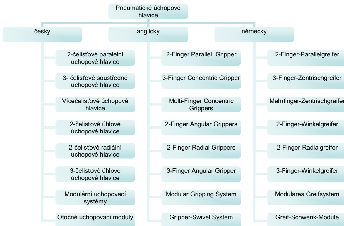
Diagram 5-8.: Pneumatické úchopové hlavice [32]
