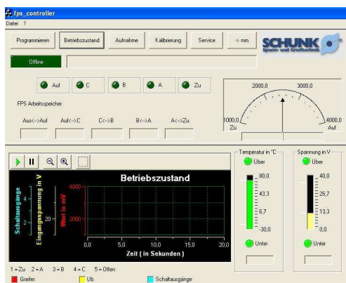
Obr. 9-15.: Příslušenství SCHUNK pro řízení chapadla MEG 64 EC [32]
