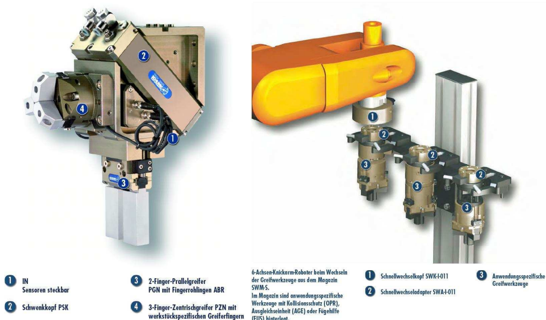
Obr. 10-6.: Otočná uchopovací hlava s dvěma chapadly [32] - vlevo
