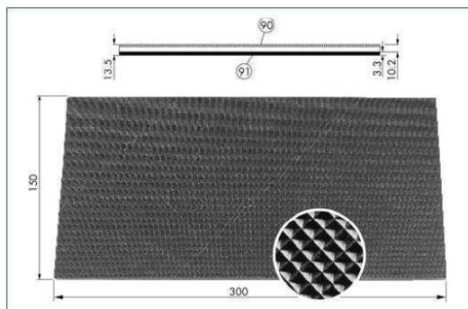
Obr. 5-12.: SCHUNK elementy Quentes, elementy z tvrdokovu, výstelky HKI [32]
