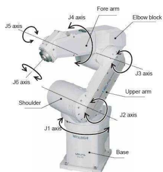
Obr. 3-1.: Rotační osy šestiosého robotu [10] - vlevo
