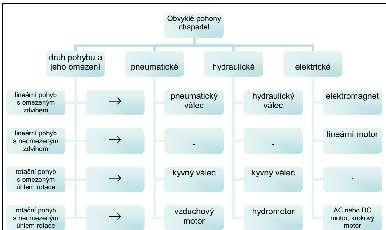
Diagram 5-4.: Obvyklé druhy pohonů chapadel podle druhu pohybu a omezení [27]
