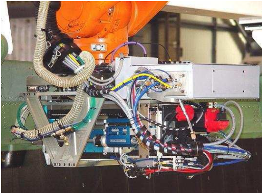
Obr. 4-6.: Multifunkční hlavice [73] – vlevo
