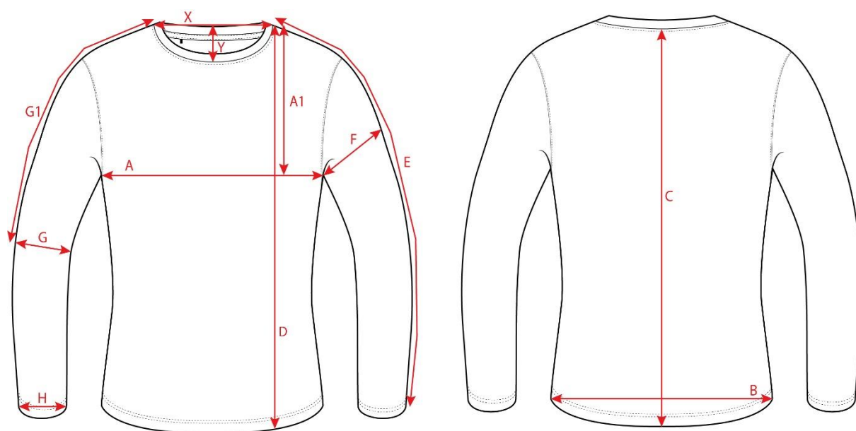
Obr. 20 Technický nákres dětského trika
