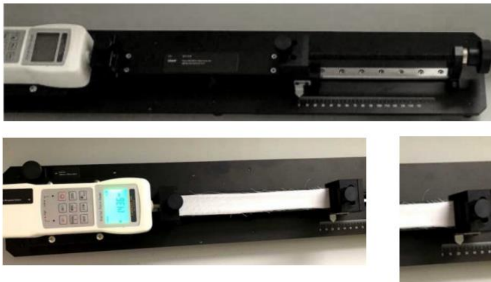
Obr.41 Měření pružnosti. [22]
