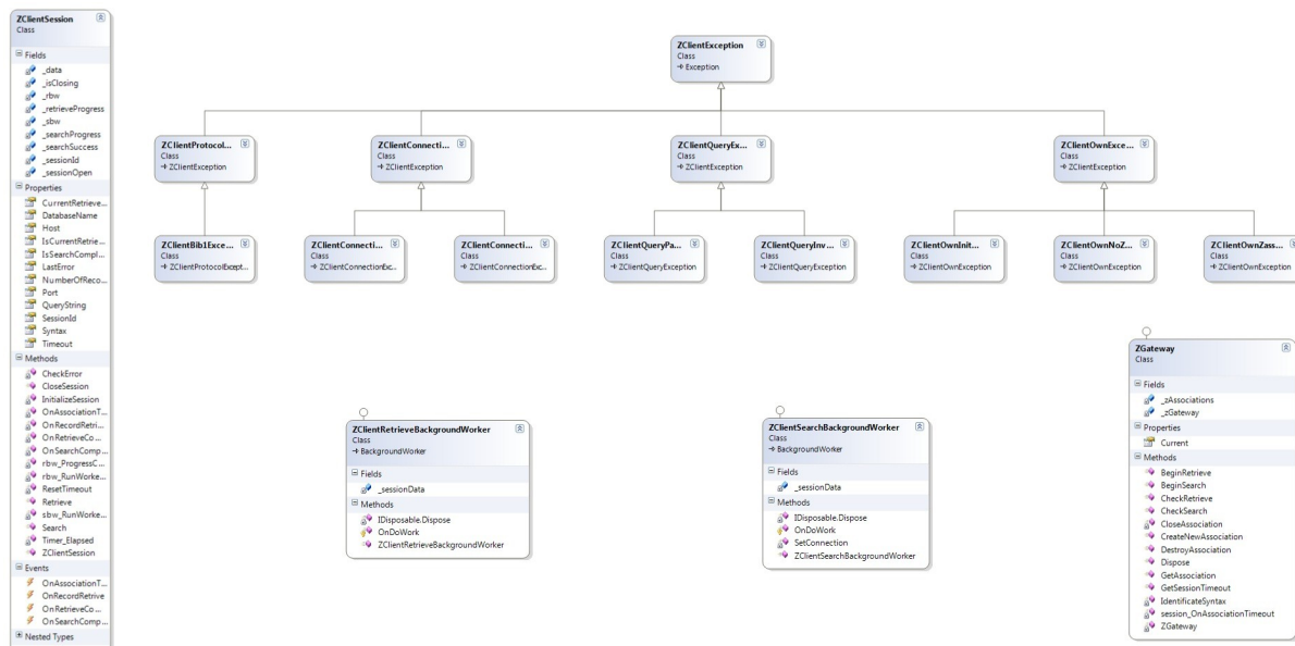
Obr.10: Diagram základních tříd Z-klienta a Z-brány.
