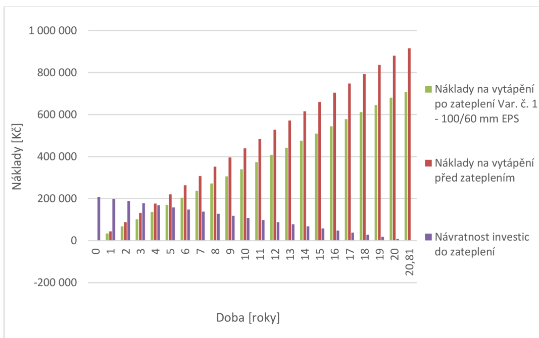
Graf. č. 6 - Návratnost investice do zateplení Var. č. 1 - 100/60 mm EPS
