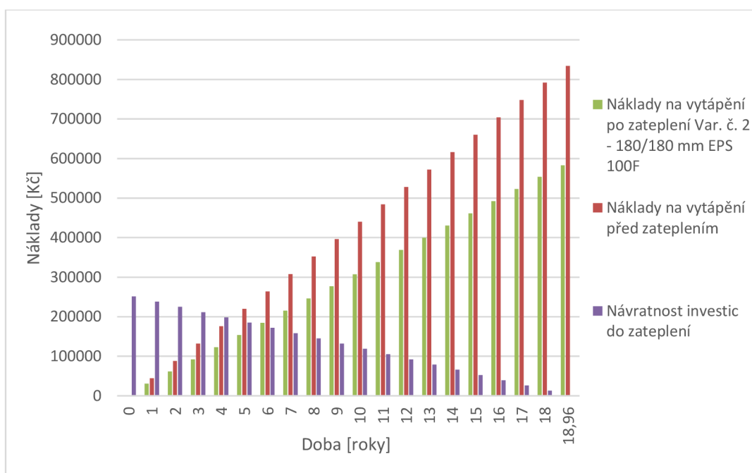
Graf. č. 7 - Návratnost investice do zateplení Var. č. 2 - 180/180 mm EPS 100F
