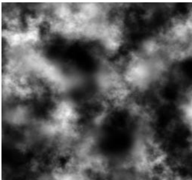
Obrázek 3- ukázka heightmapy [14]
