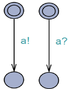
Obrázek 2.21: Synchronizační kanály v UPPAALu
