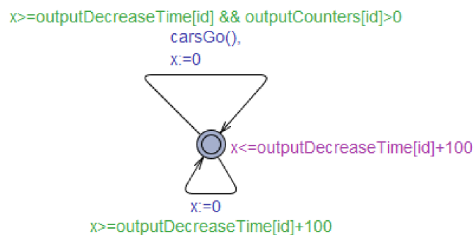
Obrázek 3.22: Automat ovládající výjezdové silnice
