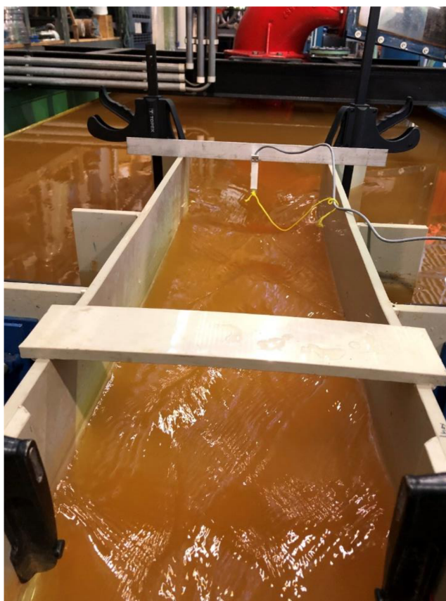
Obr. 5.15 Foto pro Q = 21 \text{ l/s}
