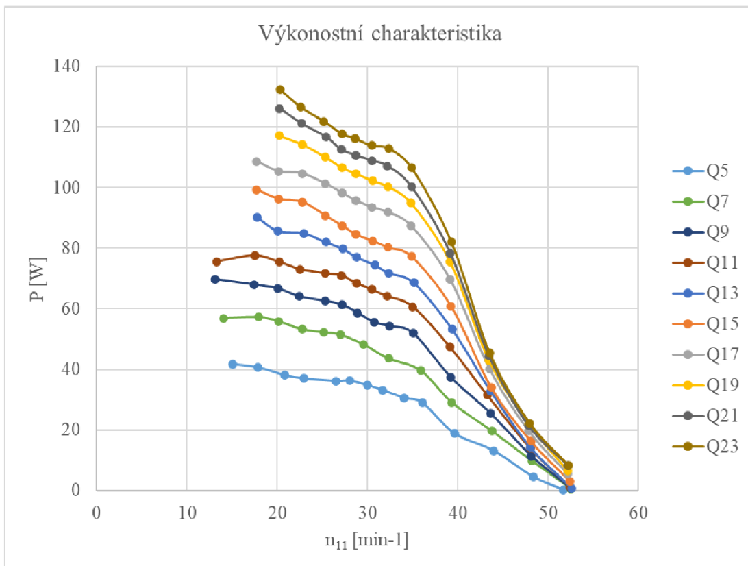
Obr. 5.10 Výkonostní charakteristika
