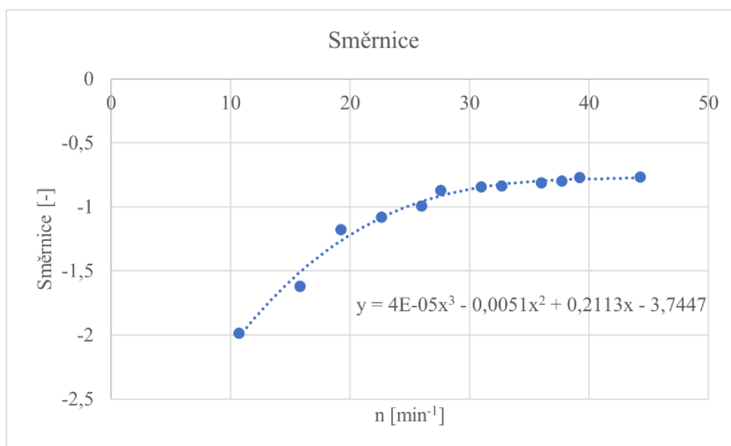
Obr. 4.5 Závislost směrnice na otáčkách
