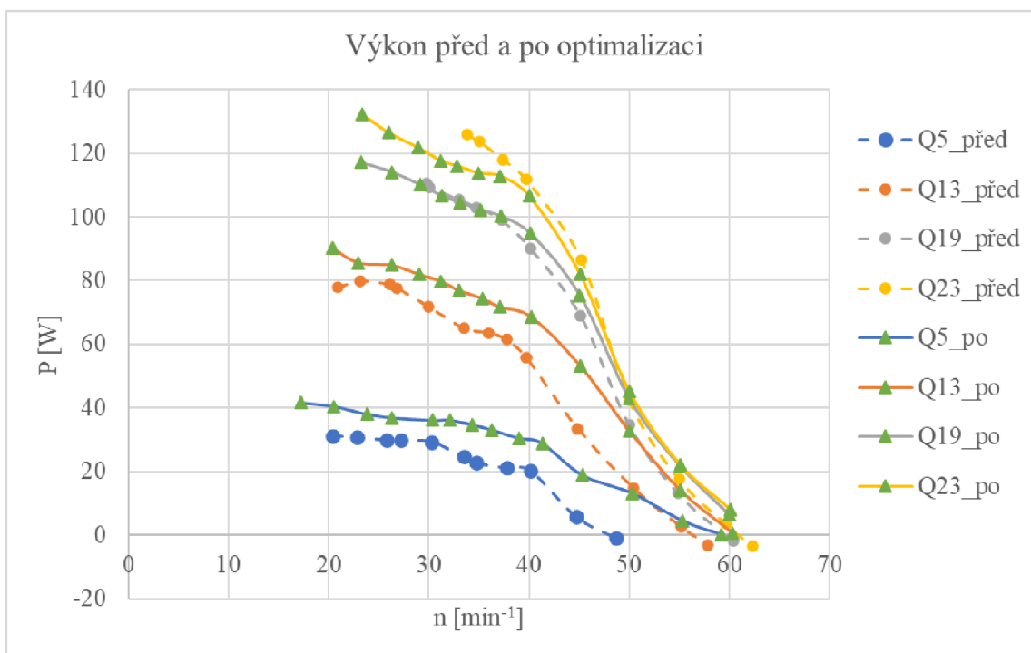
Obr. 5.19 Srovnání průběhu výkonu před a po optimalizaci
