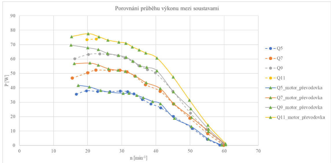
Obr. 5.4 Porovnání průběhu výkonu mezi soustavami
