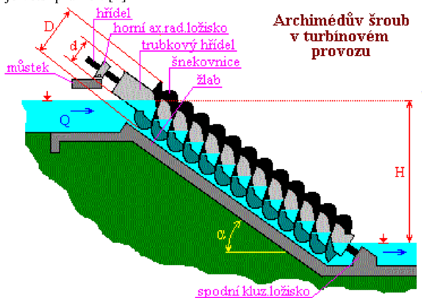
Obr. 2.2 Schéma Archimédovy turbíny [7]
