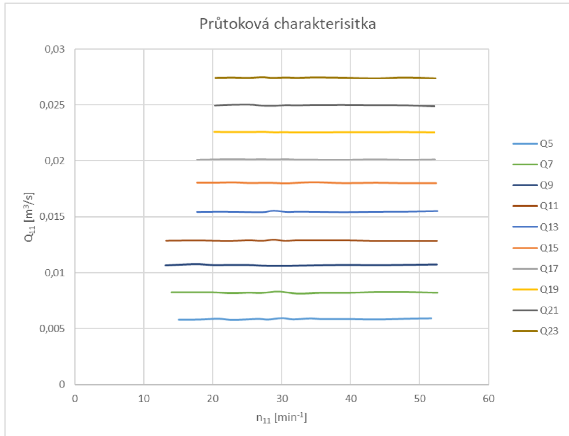
Obr. 5.8 Průtoková charakteristika
