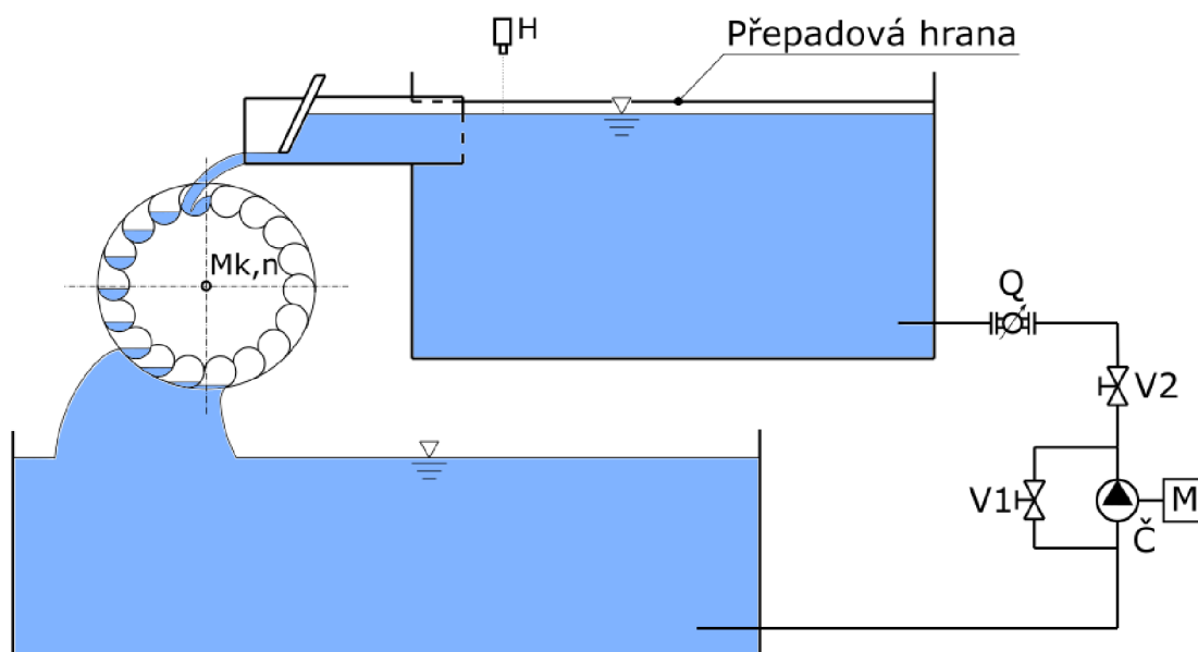
Obr. 4.1 Schéma tratě
