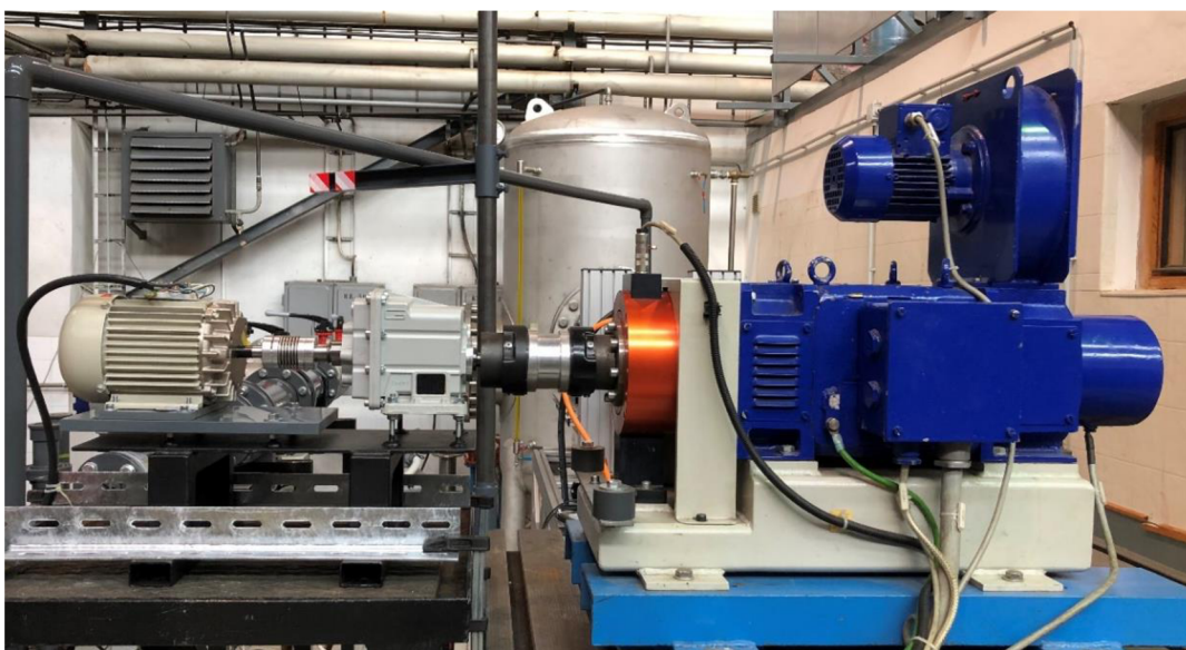
Obr. 4.2 Kalibrační soustava
