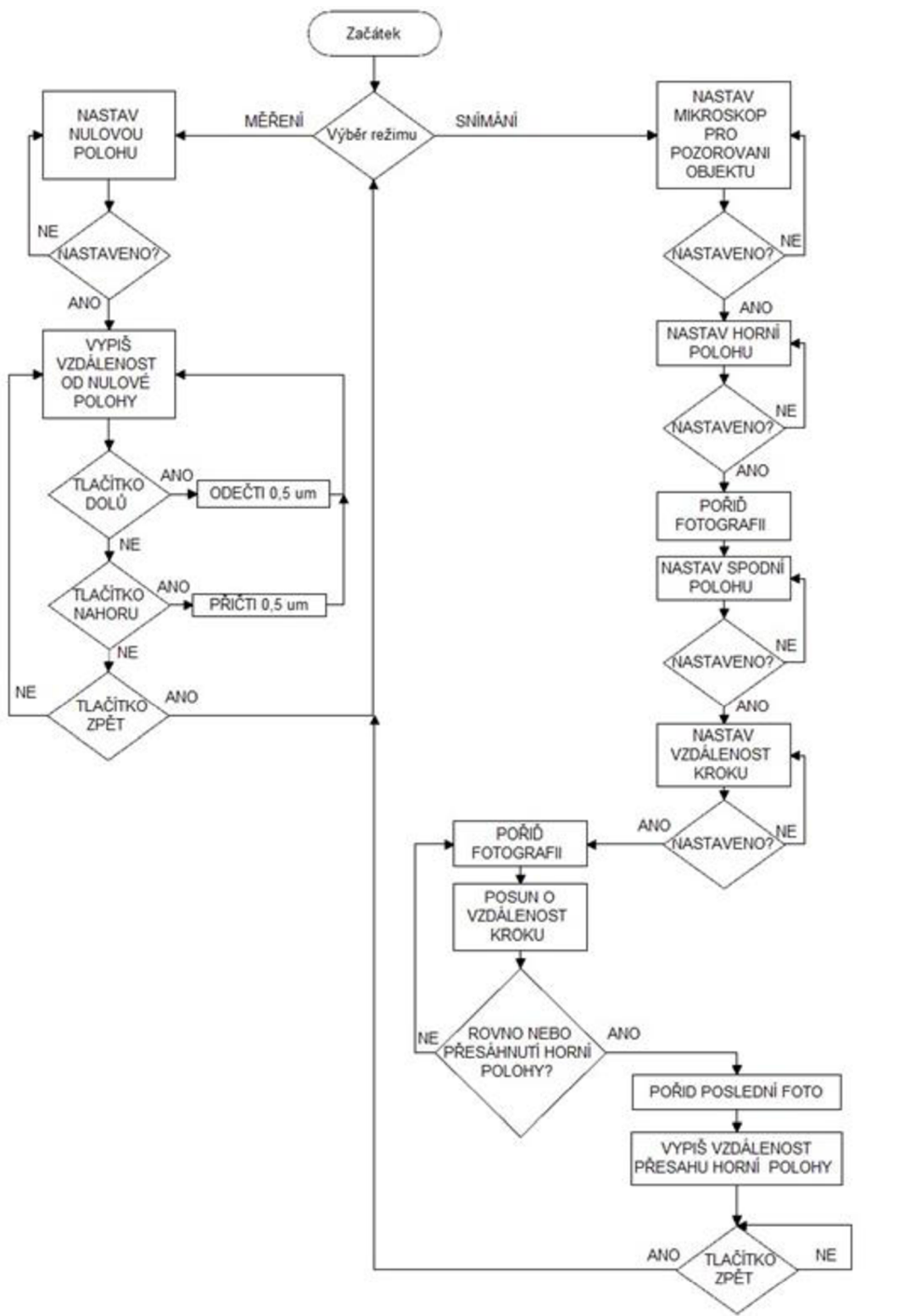
Obr. 26: Blokové schéma softwaru řídicí jednotky
