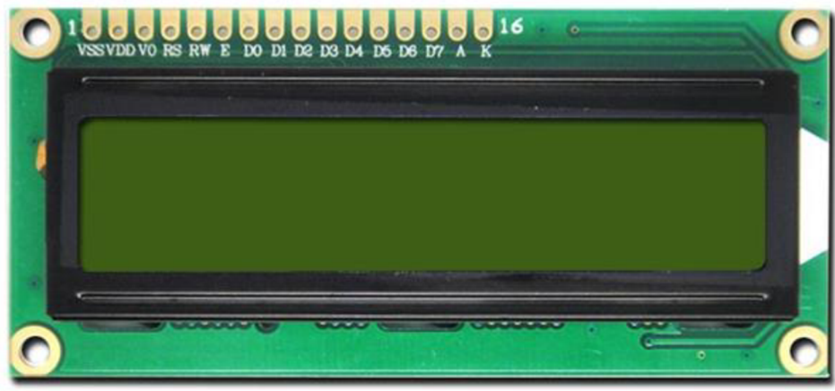
Obr. 11: Displej ATM1602B
